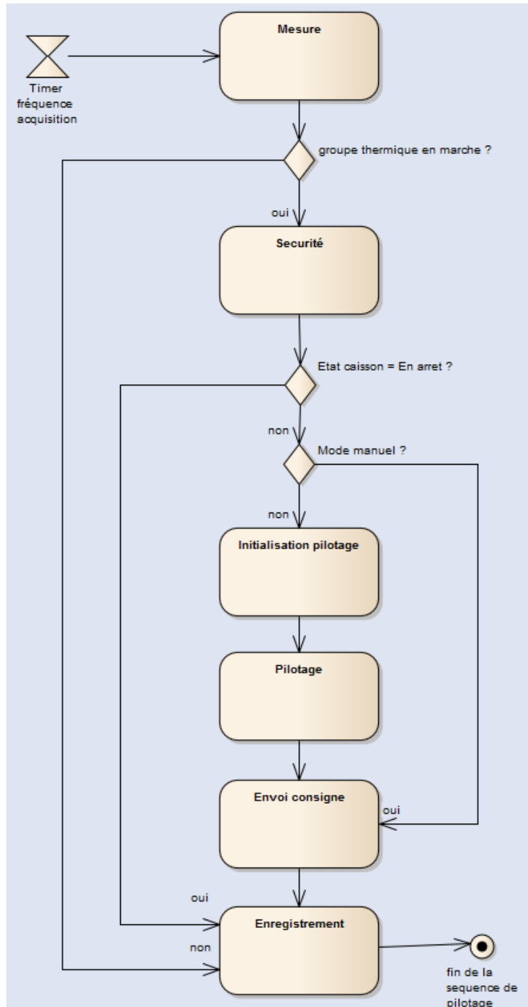
Figure 31 Diagramme d'activité pilotage
