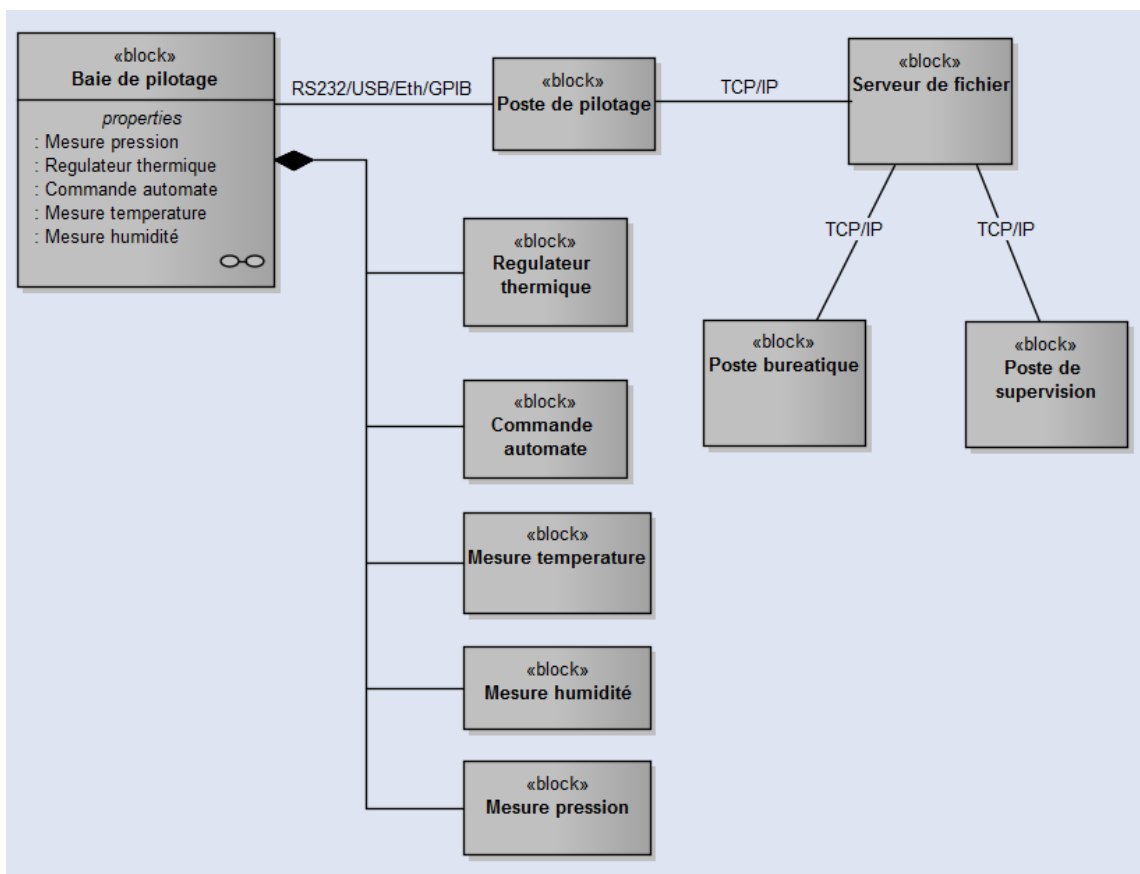
Figure 10 Diagramme de blocs composants matériels existants
