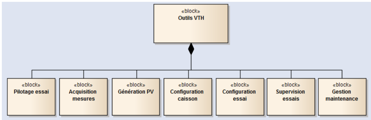
Figure 13 Architecture fonctionnelle globale
