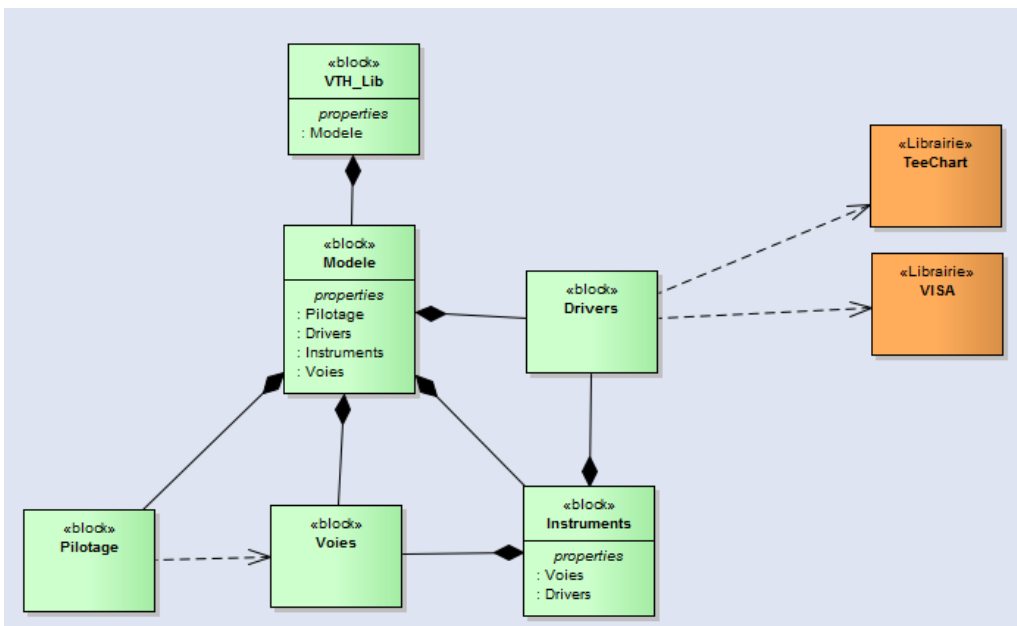
Figure 26 Compositions du modèle
