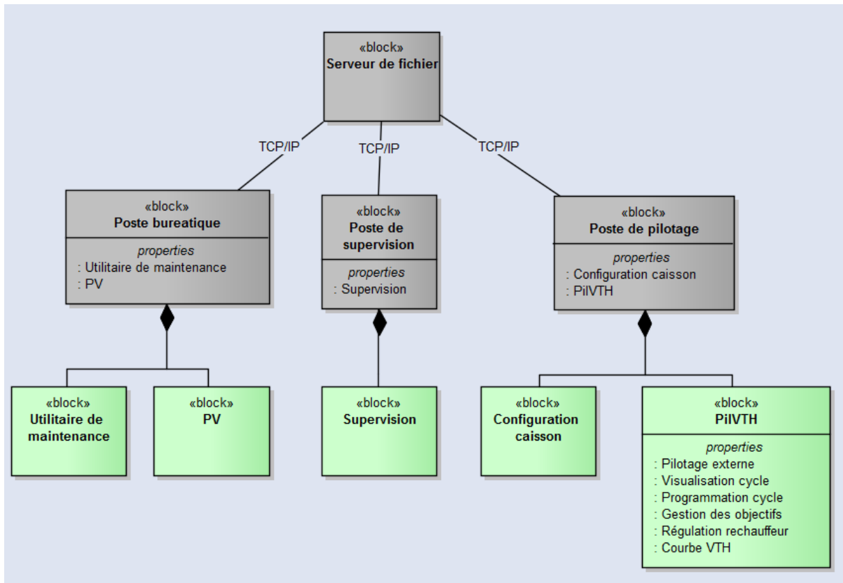
Figure 12 Architecture physique de l'existant
