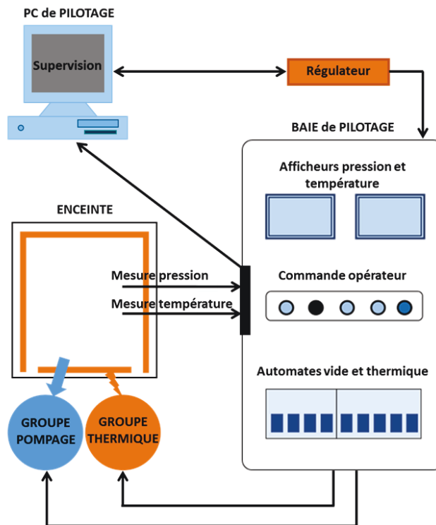
Figure 4 Schéma d'illustration d'un moyen d'essais thermique
