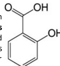
Acide salicylique
