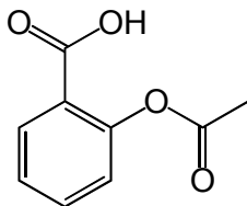
Acide acétylsalicylique
