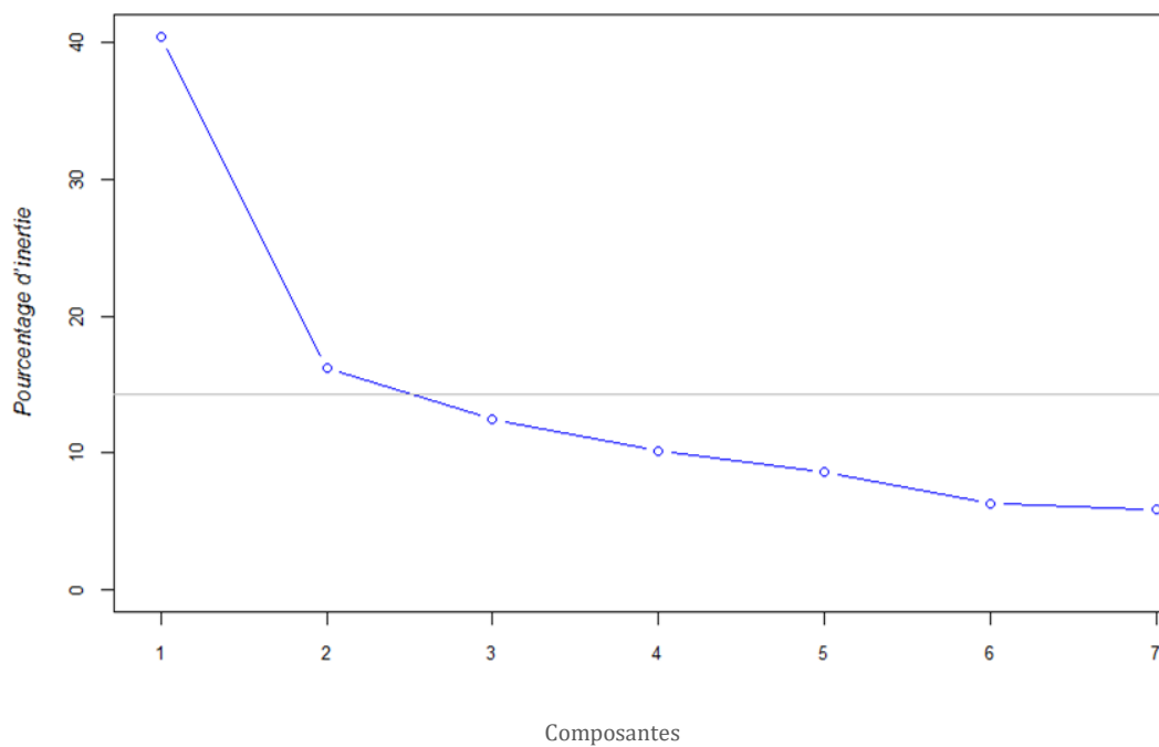
Figure 7 : Diagramme des valeurs propres
