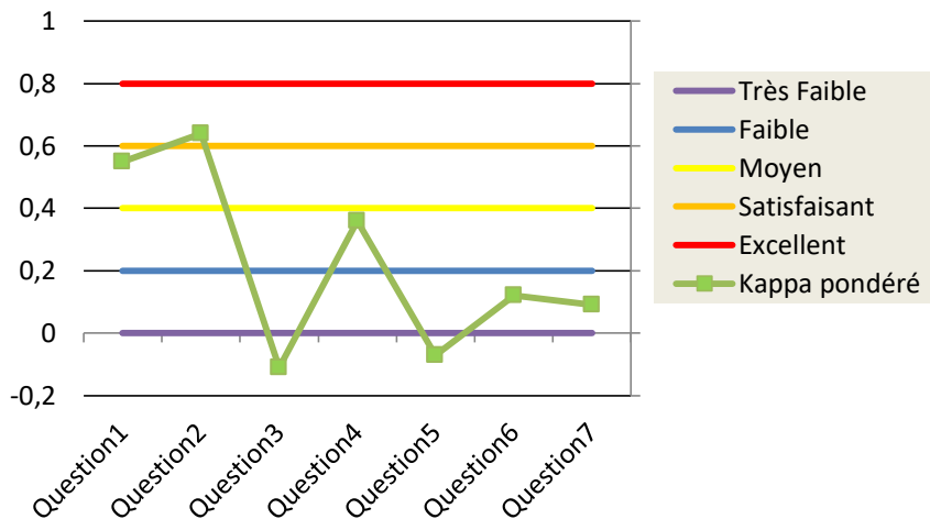
Figure 4 : Fidélité Test-Retest- Coefficient Kappa Pondéré
