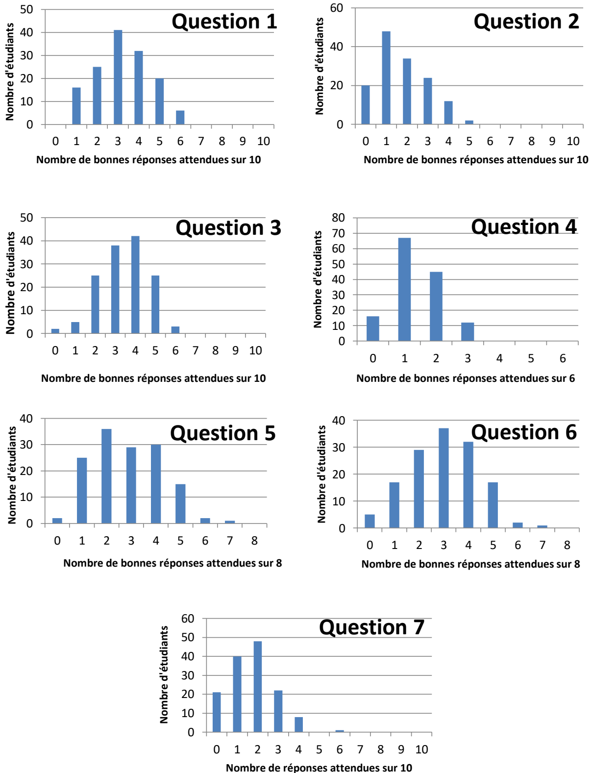
Figure 2 : Diagramme de l'effet plancher-plafond des questions 1 à 7 Page 57 sur 107
