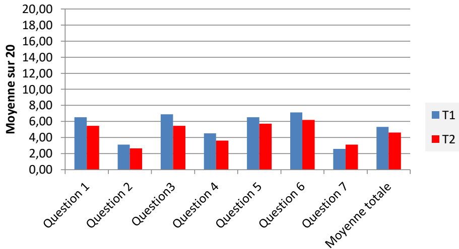
Figure 3 : Fidélité Test-Retest- Moyennes sur 20 du groupe Témoin au Test 1 et 2
