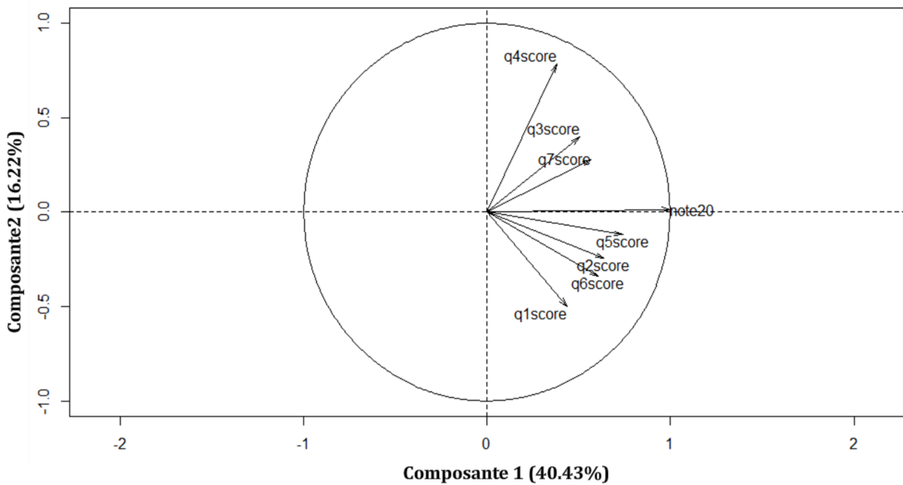
Figure 8: Graphique des variables projetées selon les deux composantes principales
