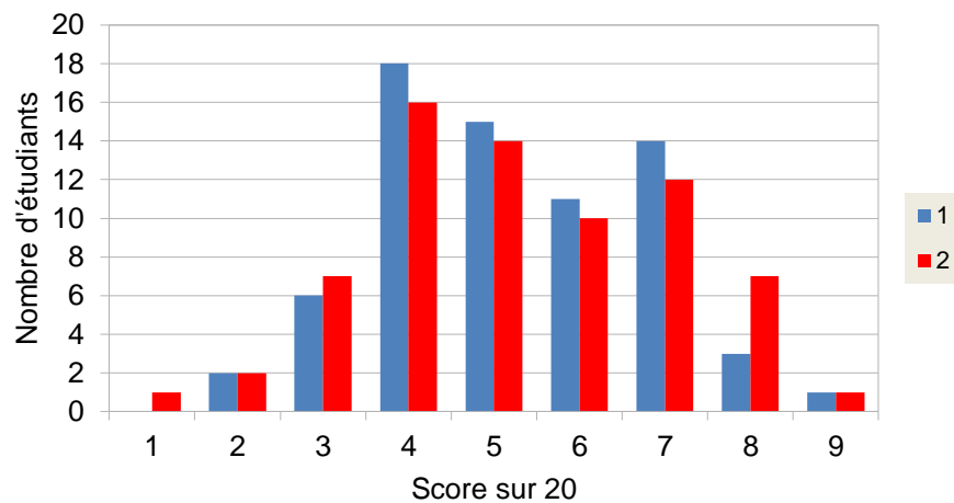
Figure 5 : Fidélité Inter Juge - Comparaison de la notation entre les juges
