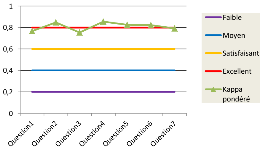
Figure 6 : Fidélité Inter Juge - Coefficient Kappa pondéré
