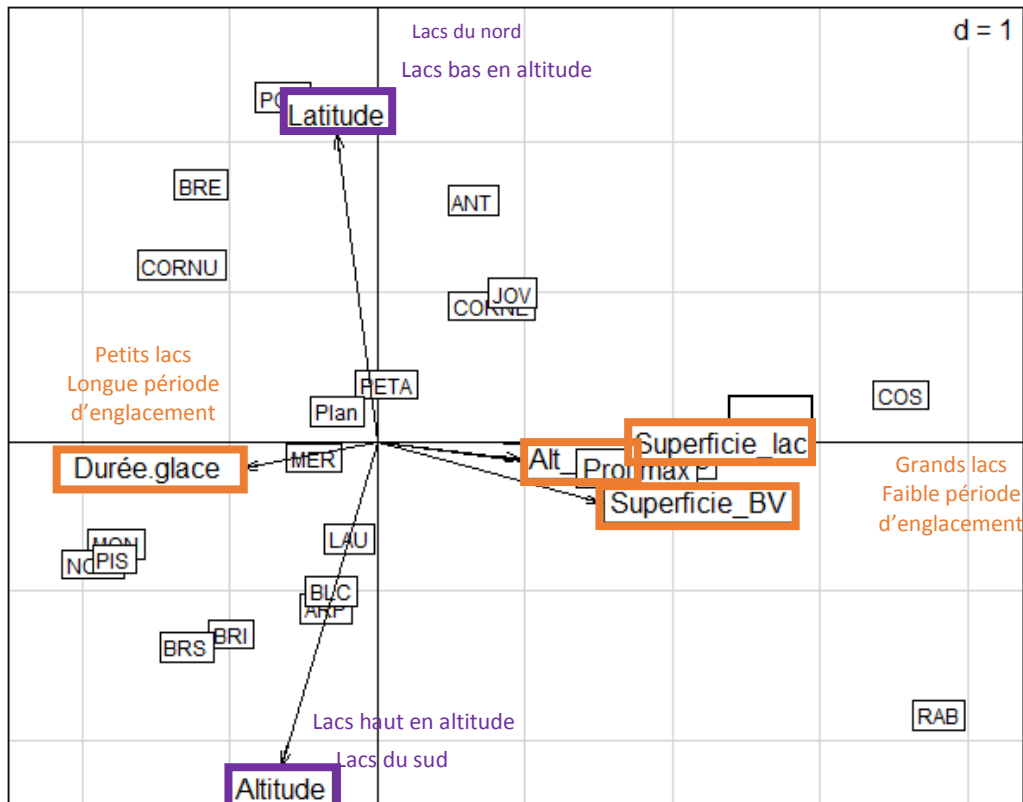
Figure 16: Résultat de l'ACP sur la morphologie et la localisation des lacs (axe 1 et 3)
