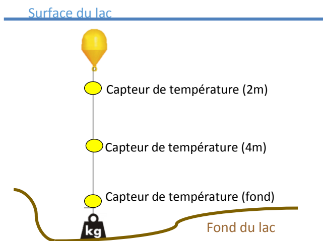
Figure 11: Disposition des capteurs de température permanents dans les lacs
