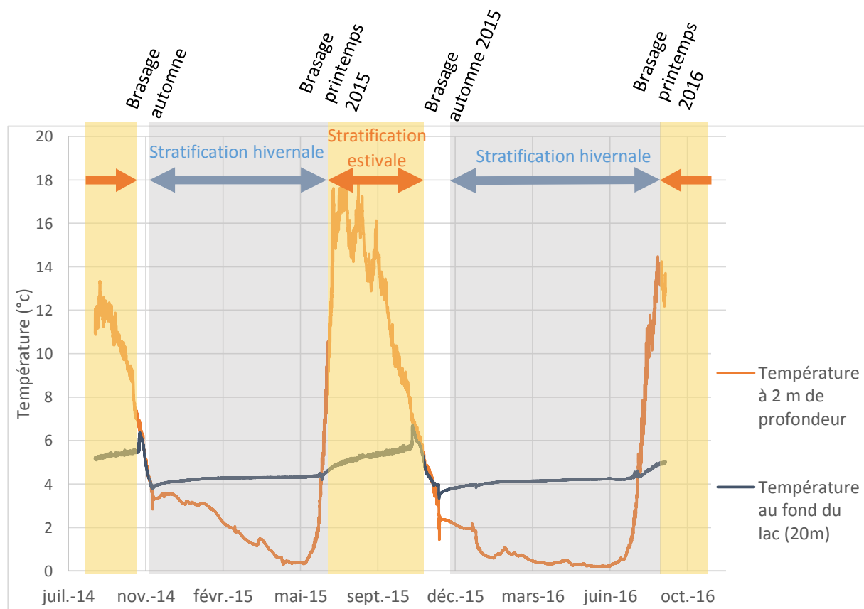
Figure 4 : Evolution des températures de surface et du fond du lac Cornu entre septembre 2014 et septembre 2016
