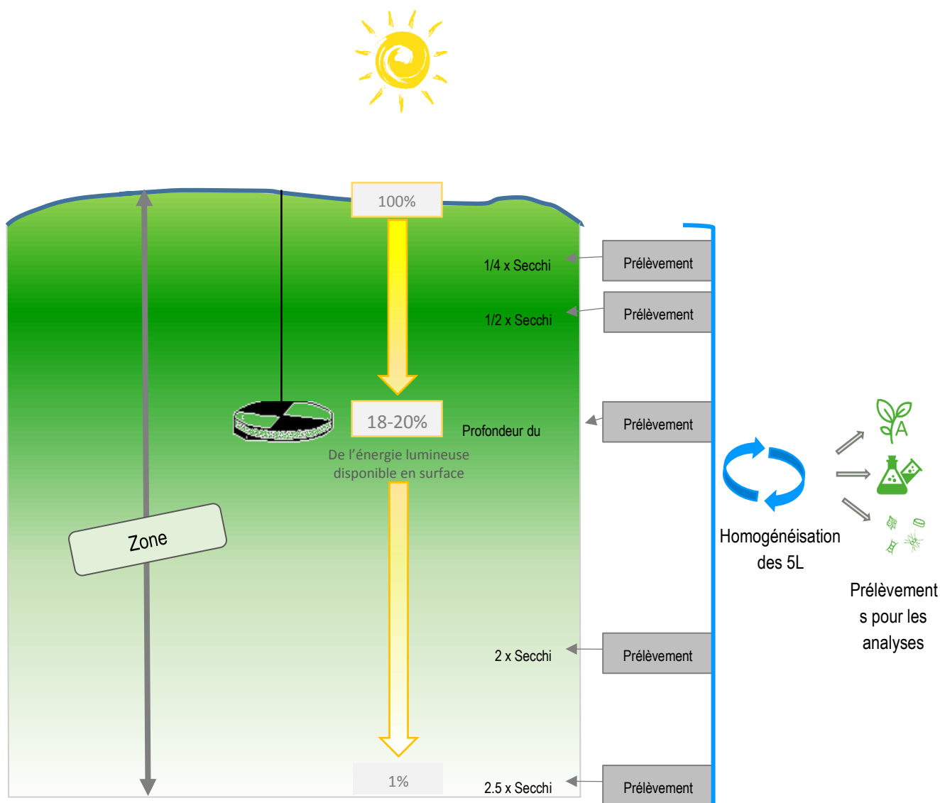
Figure 4 : Nouveau protocole proposé pour le prélèvement en surface
