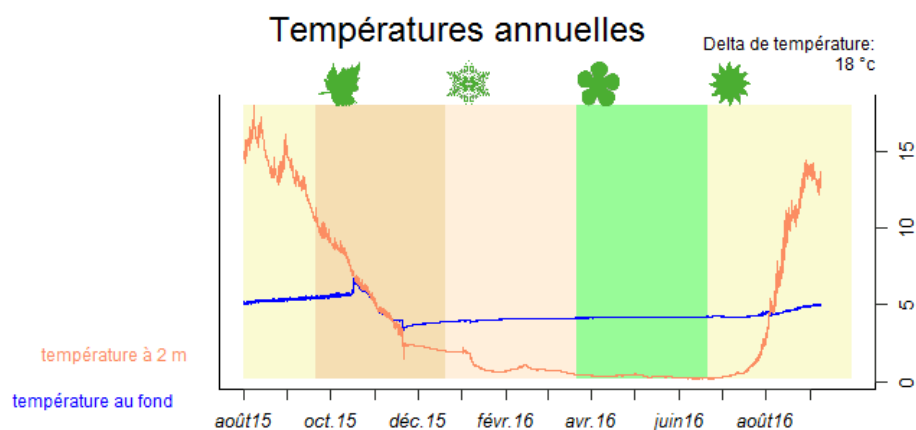
Figure 14: Graphique présenté dans la fiche lac, évolution des températures du lac de Corne entre septembre 2015 et septembre 2016
