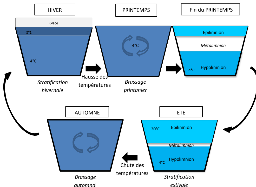
Figure 5: Evolution des différentes couches d'un lac dimictique dans l'année
