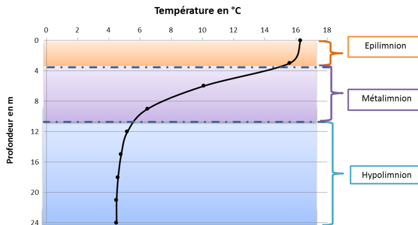
Figure 3: Evolution de la température dans un lac selon la profondeur (PiburgerSee, juin 2015)
