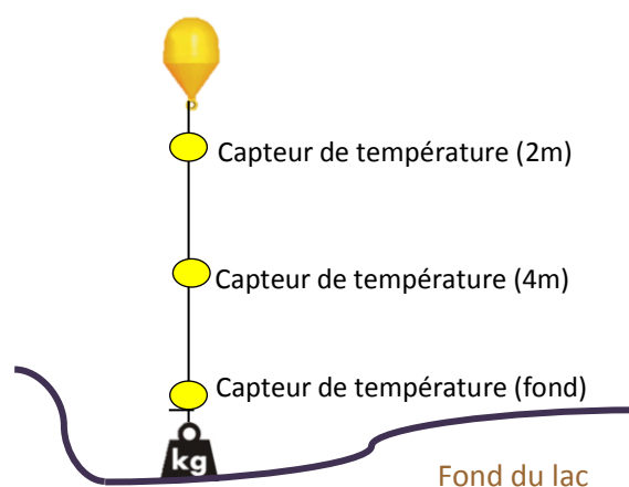
Figure 1: Disposition des capteurs de température permanents dans les lacs
