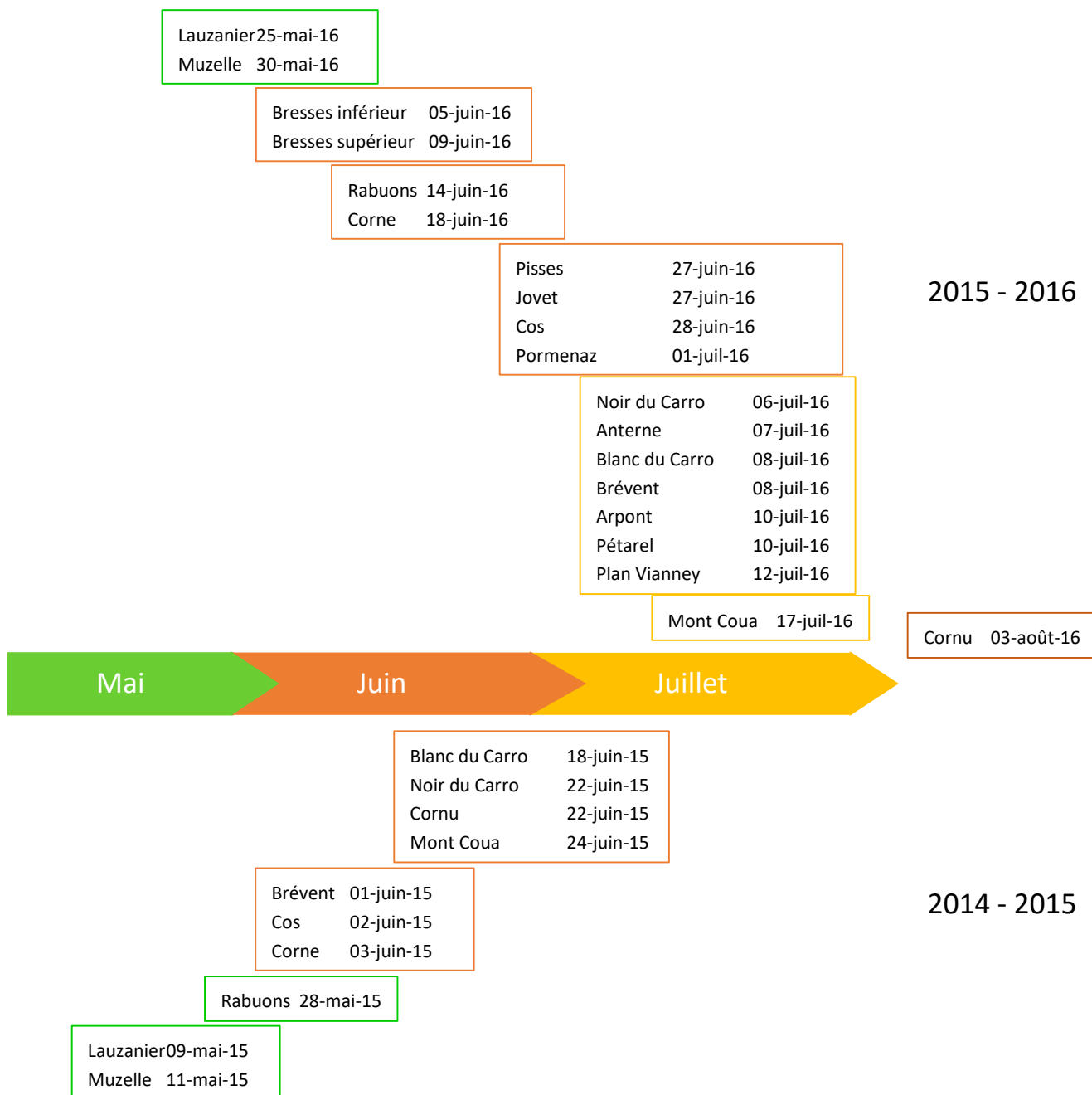
Figure D: Frise résumant les dates de déprise en glace pour les deux années
