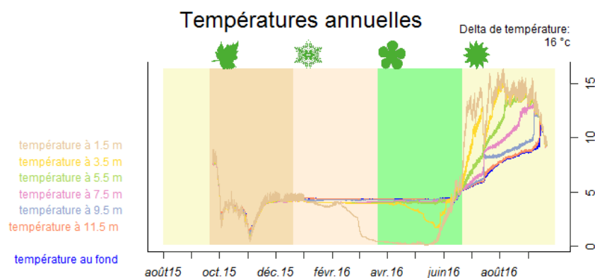
Figure B: Evolution des températures entre septembre 2015 et septembre 2016, lac de Bresses supérieur
