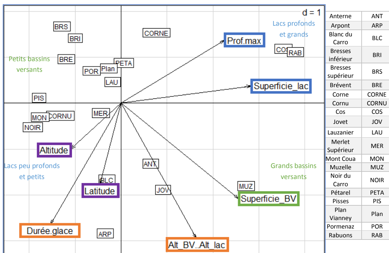
Figure 15: Résultat de l'ACP sur la morphologie et la localisation des lacs (axe 1 et 2)
