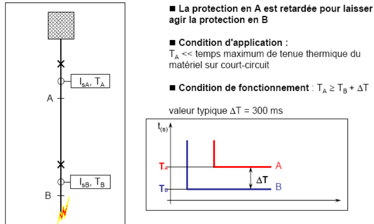
Figure 17: Sélectivité chronométrique
