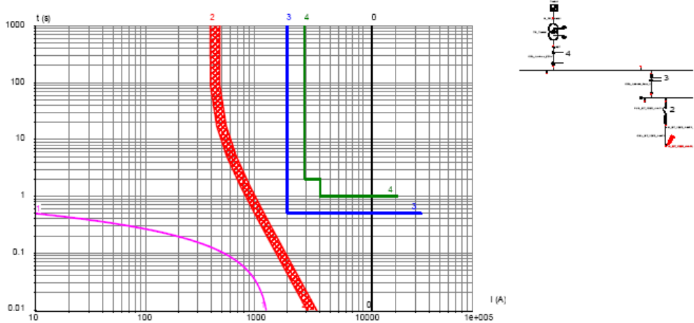
Graphique de coordination des protections
