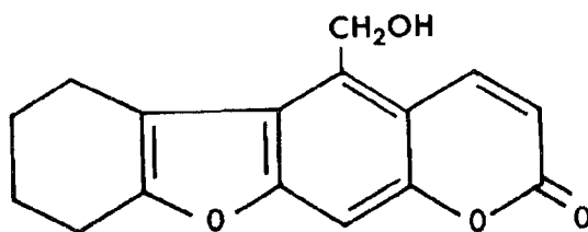
benzoangélicine
