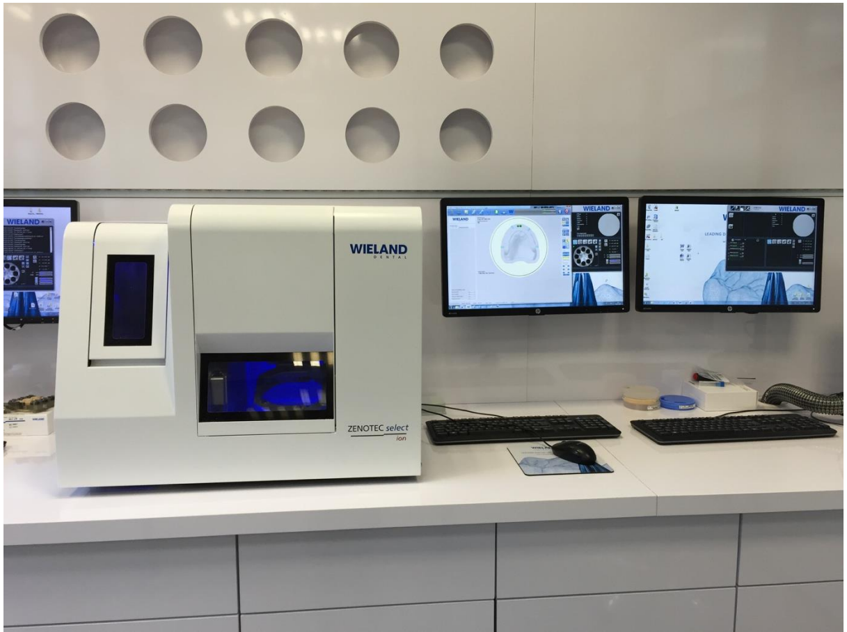
Figure 53 : Usineuse – Fraiseuse
