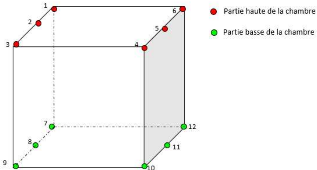
Figure 22. Schéma de l'emplacement des indicateurs biologiques
