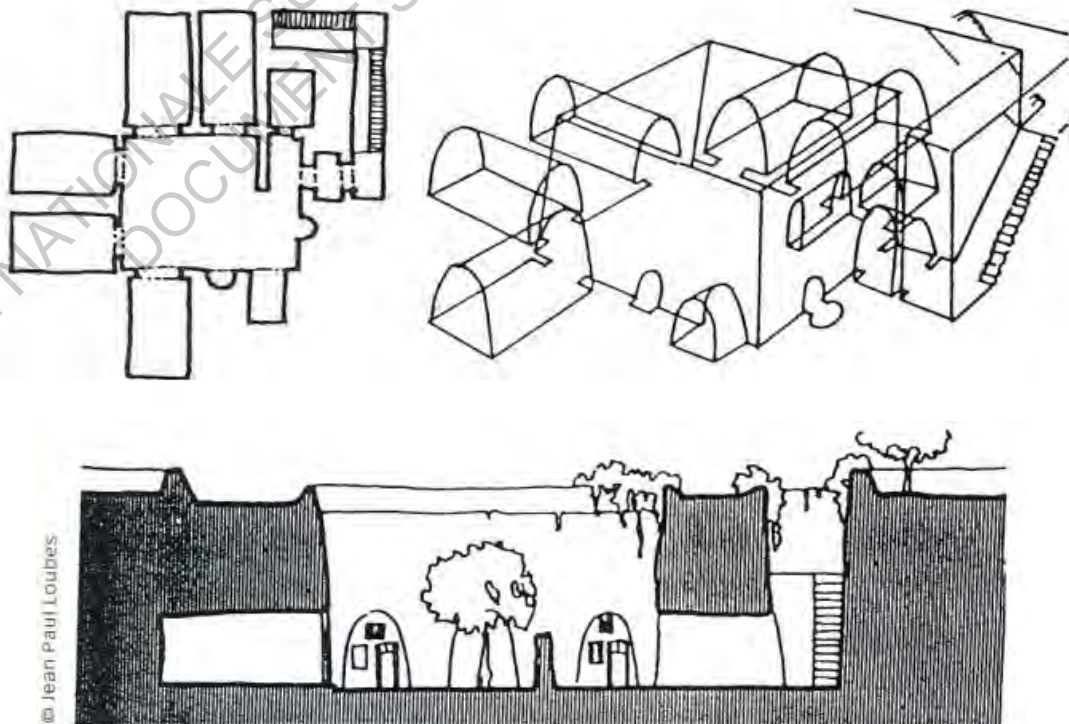
Plan, coupe, et , axonomie d'une maison troglodytique (tianjing yuan shi) Gansu
