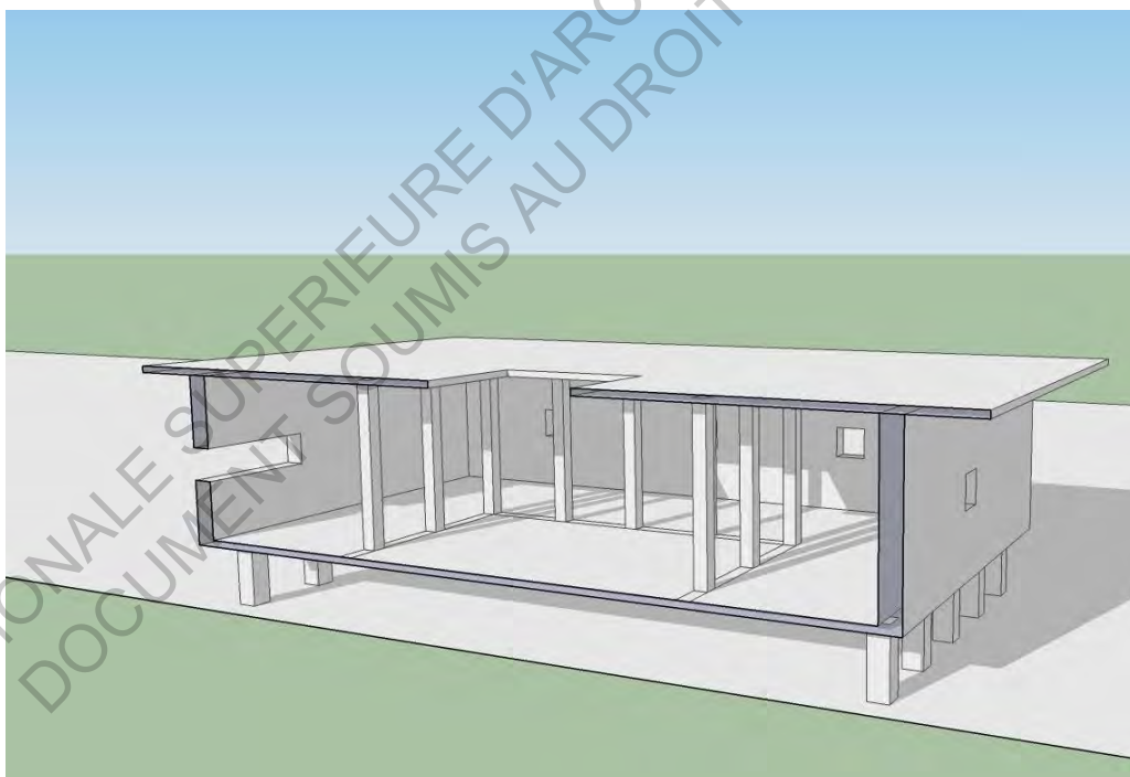
Photographie : WeekEnd House Ryū Nishizawa(Japon) 1998 Et modélisation d'un exemple de dispositif type
