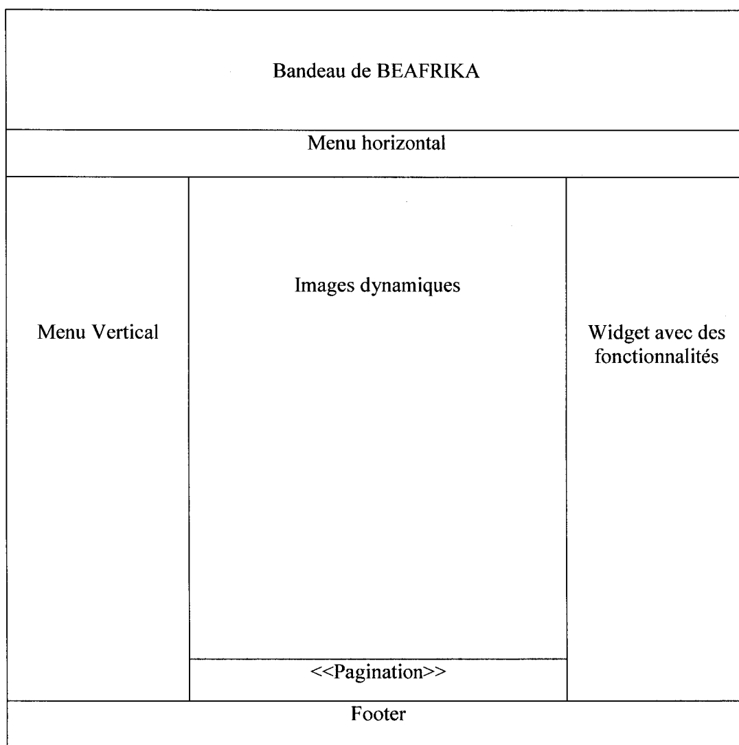
Figure 2 Architecture des pages catégories(Articles)
