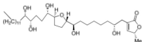
annopentocin B
