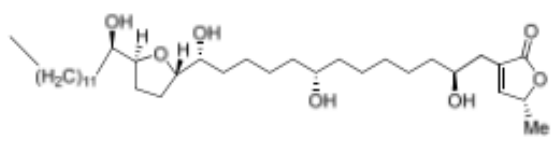
annonacin A
