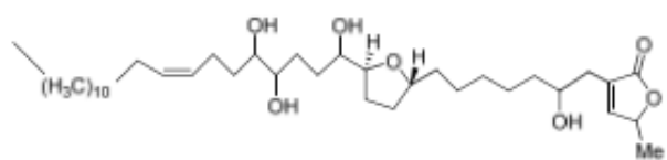
gigantetronenin
