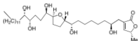
annopentocin A
