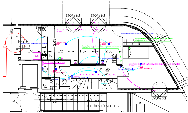
FIGURE A.2 – Premier étage de l'appartement Amiqua4Home
