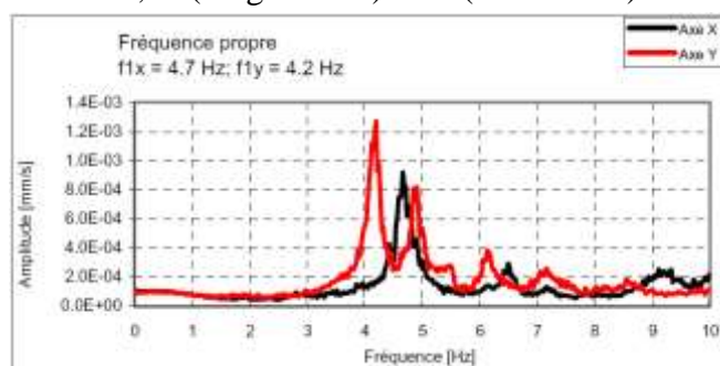
Figure 2.4.2: Exemple de graphe des fréquences donnée par l'appareil d'acquisition pour un bâtiment..
