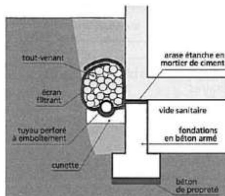
Figure 4.4.5 : Drainage périphérique.
