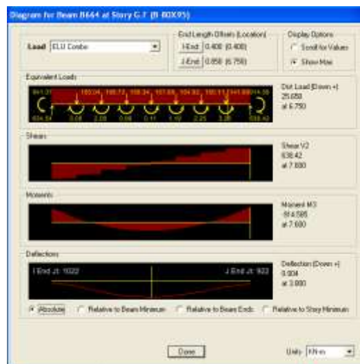
Figure 6.3.2 : Les efforts agissant sur la poutre choisi, selon ETABS.
