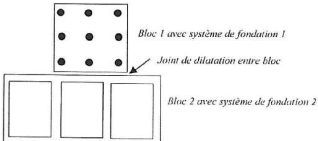
Figure 4.4.3 : Exemple de système de fondation hétérogène (mais acceptable car séparé).
