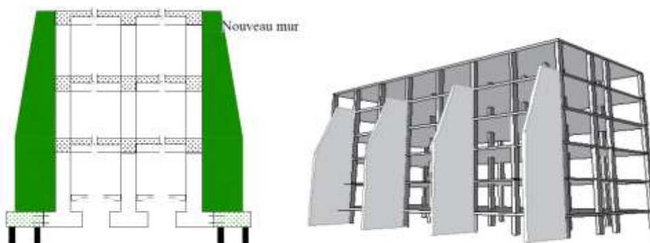
Figure 3.3.15 : Schéma en 2D et 3D des murs de contreforts à l'extérieur.
