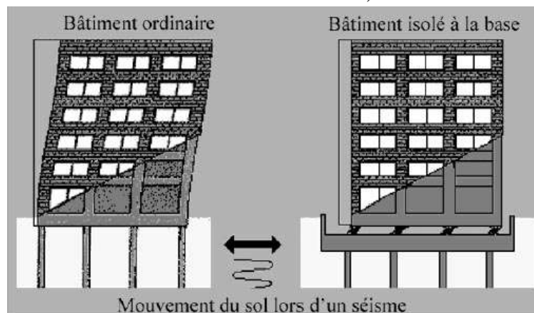
Figure 3.1.1 : Mouvement d'un bâtiment ordinaire et un autre isolé lors d'un séisme.
