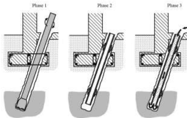
Figure 3.4.6 : Schéma des étapes d'installation des micro pieux.
