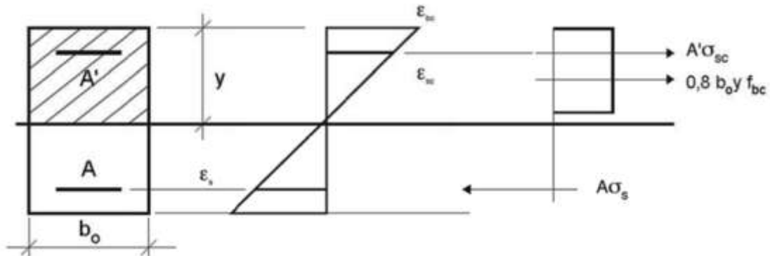
Figure 3.3.1 : Diagramme De contrainte en ELU d'une section poutre.
