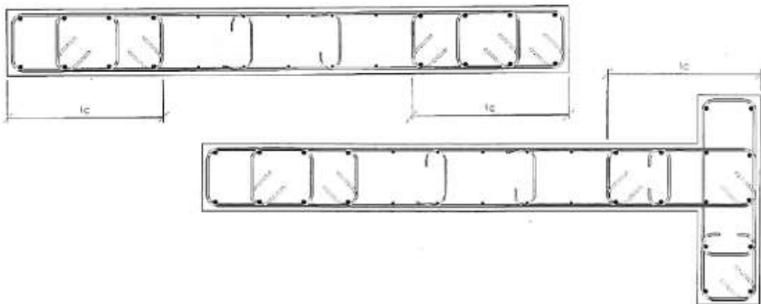
Figure 4.4.2 : Schéma de ferrailage des murs représentant l_c .
