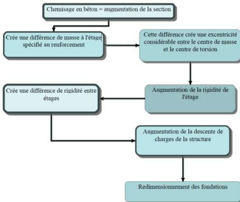
Figure 3.3.5 : Organigramme du processus de chemisage en béton armé.
