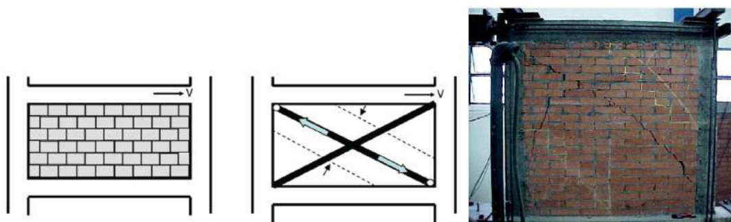
Figure 3.3.16 : Schéma d'un mur de remplissage et son mode de rupture.
