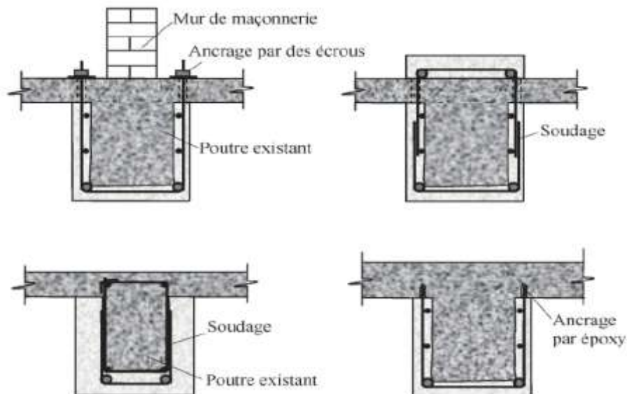
Figure 3.3.2 : Schéma des chemisages d'une poutre en béton armé.
