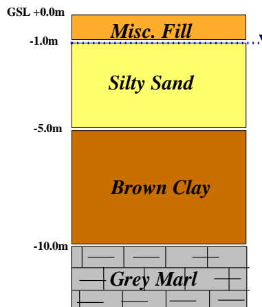
Figure 5.1.11 : Profile du sous-sol.
