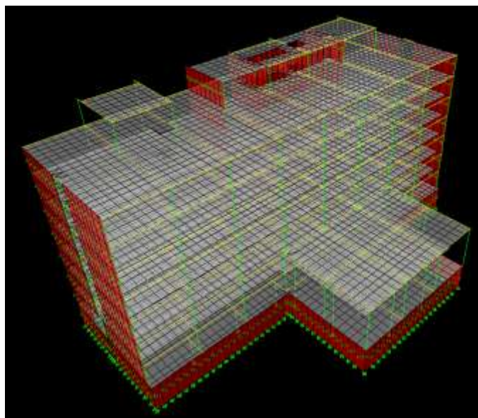
Figure 7.1.1 : Image en 3D du bâtiment renforcé.
