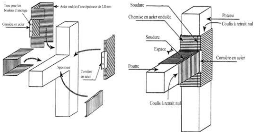
Figure 3.3.7 : Schéma d'assemblage de chemise d'un nœud poutre-poteau.
