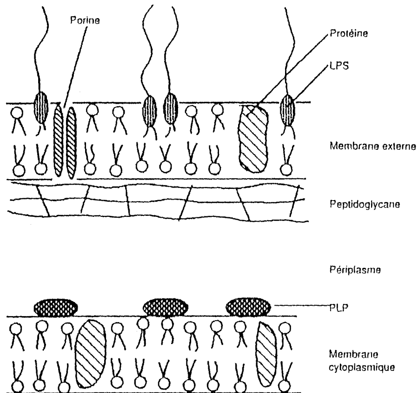
Fig 2: structure de la paroi des bactéries Gram négatif
