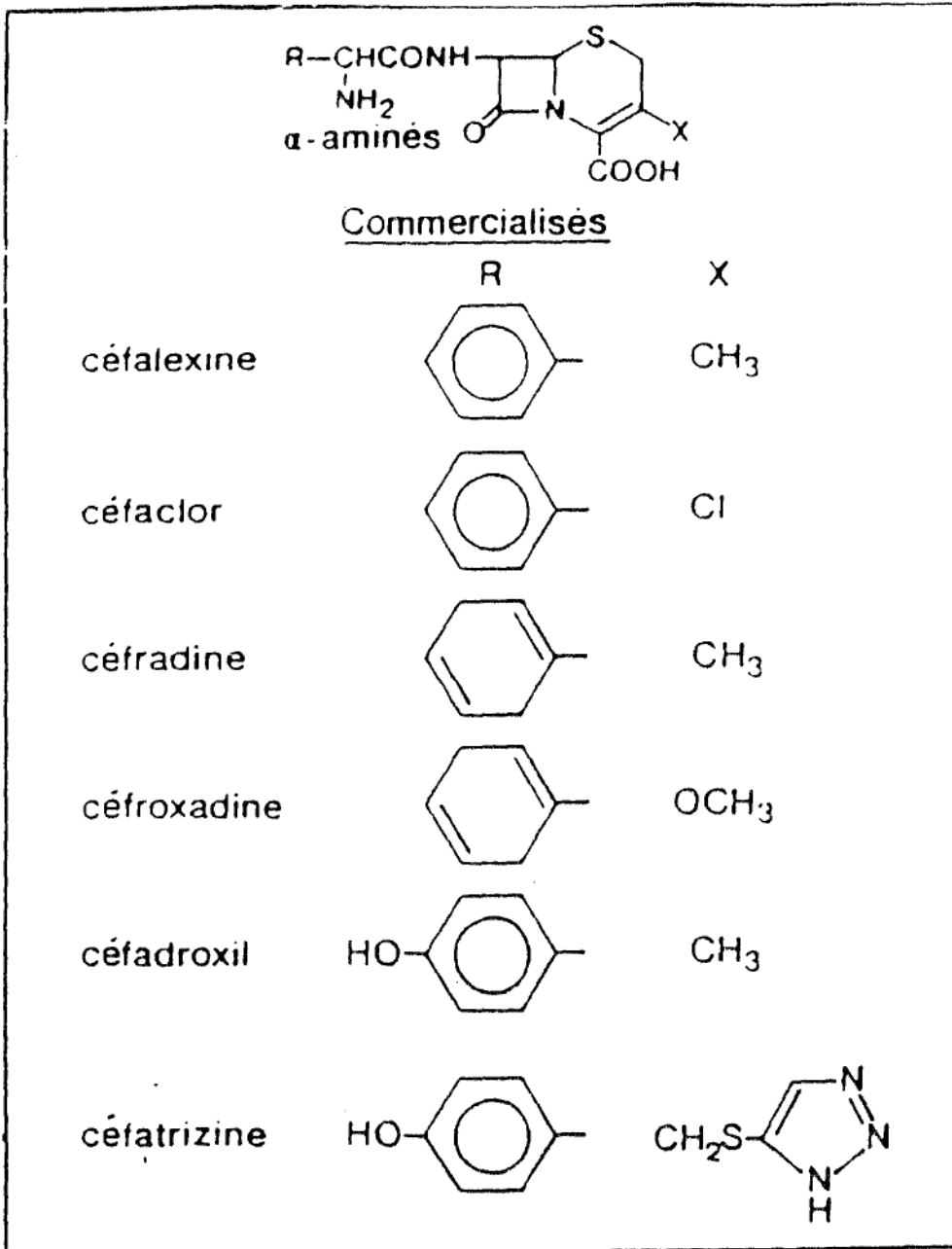
Structures des céphalosporines de première génération
