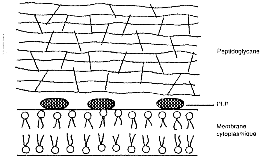
Fig 1: structure de la paroi des bactéries Gram positif
