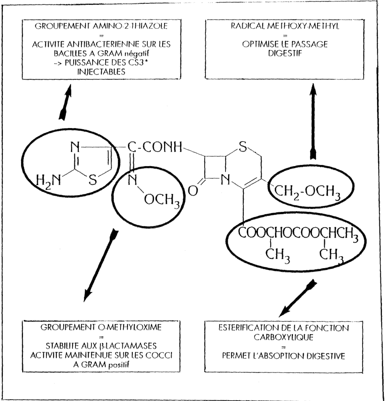
Structure du céfpodoxime proxétel
