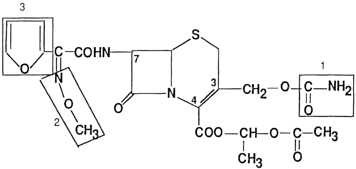
Structure de céfuroxime axétil
