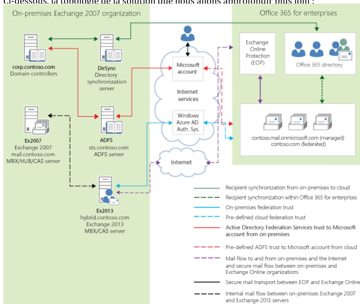
Figure 6: topologie de la solution hybride proposée au client
