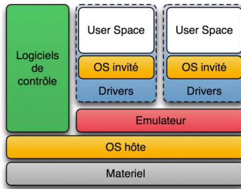
Figure 9 La virtualisation de niveau 2 (source wikipedia)
