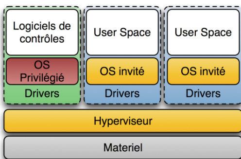
Figure 8 La virtualisation de niveau 1 (source wikipedia)
