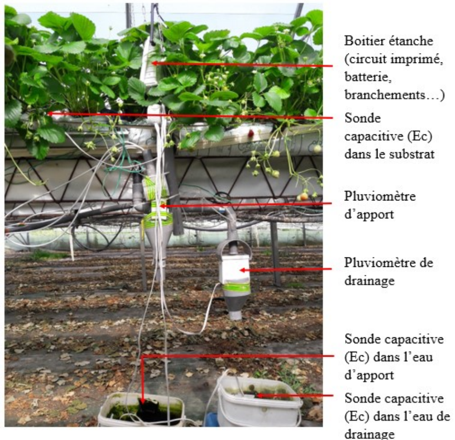
Figure 6 : vue de l'outil récupérateur de données installé sur la parcelle 3 avec les deux sondes capacitatives dans des seaux. Les autres parcelles sont équipées avec des siphons permettant aux sondes de toujours être en contact avec l'eau (photographie prise le 15/05/2018 dans le Val de Caudeau Louyre, par Léa Zerbino)
