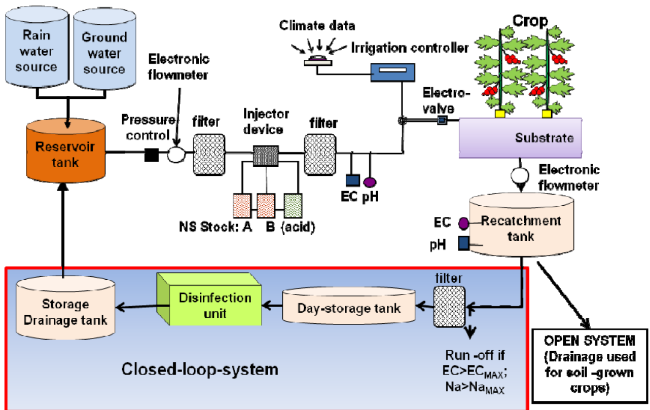
Figure 3 : schéma d'une installation type pour une production hors-sol en circuit ouvert ou fermé (Pardossi et al., 2011)
