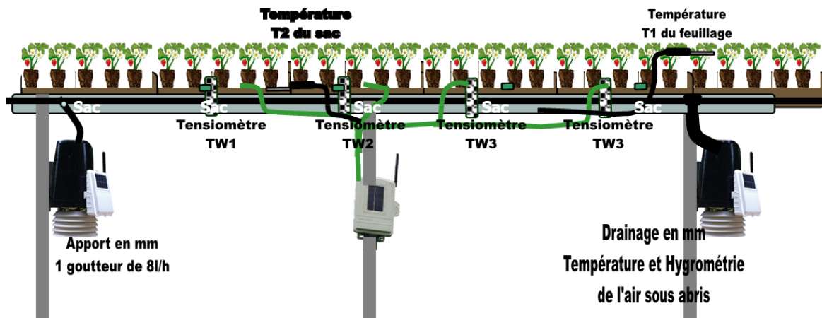
Figure 5 : Schéma de la station de récupération de données sur la parcelle 3 ; les parcelles 1, 2 et 4 ne possèdent pas de tensiomètres, mais ont le même type d'installation (document interne, 2017)
