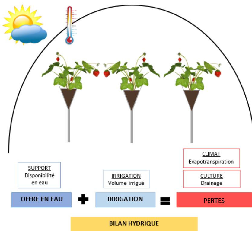
Figure 6 : schématisation de la méthode de calcul du bilan hydrique en fonction des éléments du système (Zerbino, 2018)
