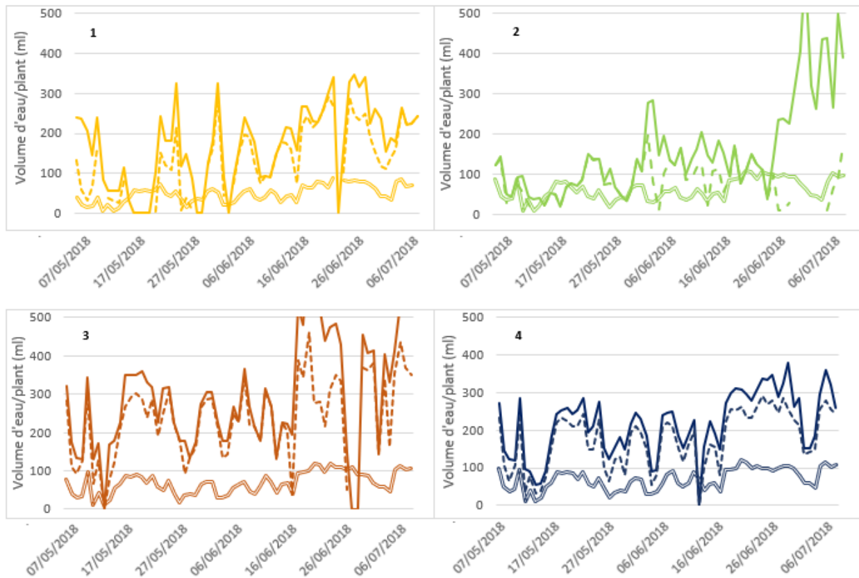
Figure 7 : évolution et comparaison des volumes apportés ( — ), volumes consommés ( - - - ), et besoins théoriques ( ⋯ ) pour les quatre parcelles sur toute la saison de production. Les valeurs hors cadre restent inférieures à 600 ml/jour pour les parcelles 2 et 3.
