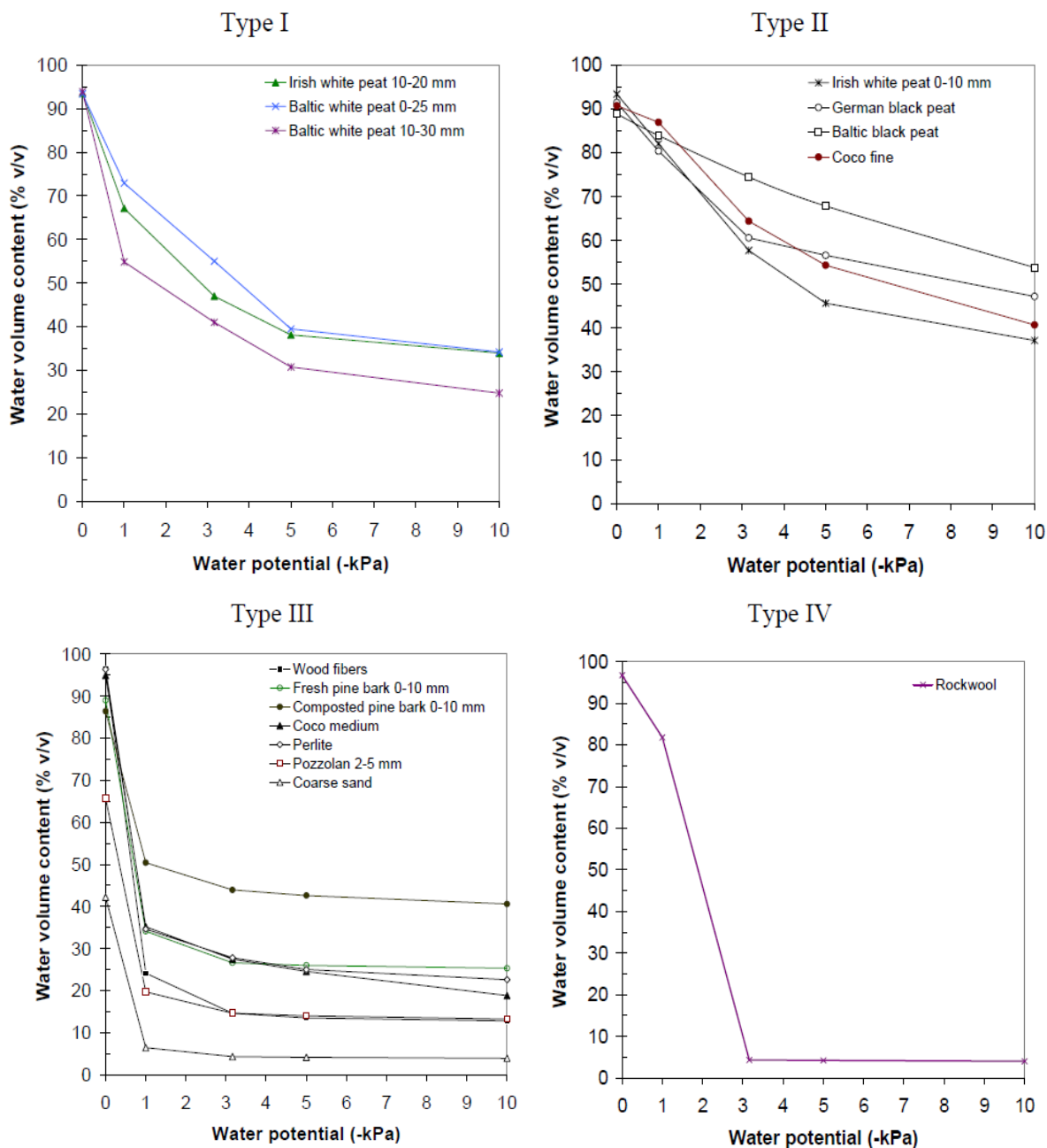
Figure 2: Exemples des types de courbes de rétention d'eau de différents matériaux utilisés comme support de culture pour le hors-sol. La production de fraises se fait essentiellement sur de l'écorce compostée, du mélange tourbe/écorce et des fibres de coco (Michel, 2010)
