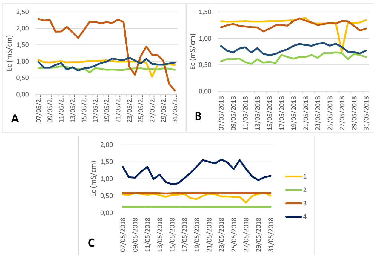
Figure 8 : évolution et comparaison des conductivités ( E_c ) sur le mois de mai à l'apport (A), dans le sac (B) et au drainage (C) pour les quatre parcelles
