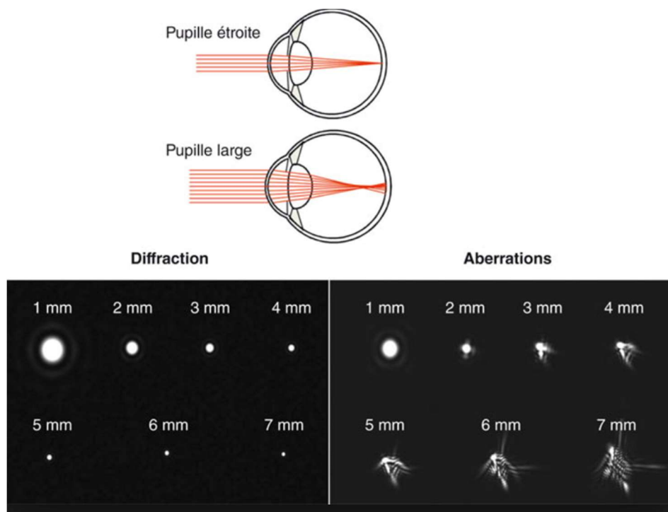
Figure 9 : Diffraction et aberration en fonction de la taille de la pupille
