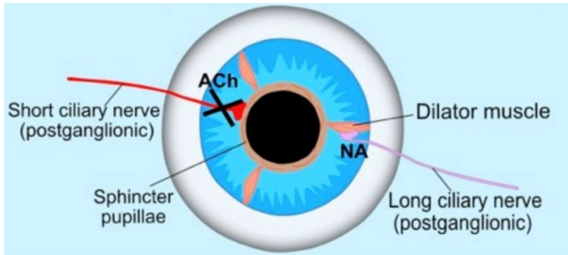
Figure 4 : La pupille et le système musculo-nerveux qui influence sa taille (Source : Hall et Al.(6))
