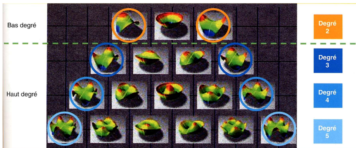
Figure 16 : Polynômes de Zernike pour l'analyse de la décomposition du front d'onde
