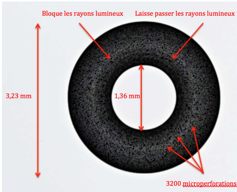
Figure 38 : Masque de carbone avec ouverture centrale incorporé au centre de la lentille
