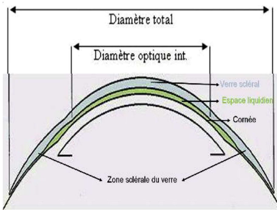
Figure 23 : Schéma de la lentille sclérale (Source : Service d'Ophtalmologie, CHU Rouen)
