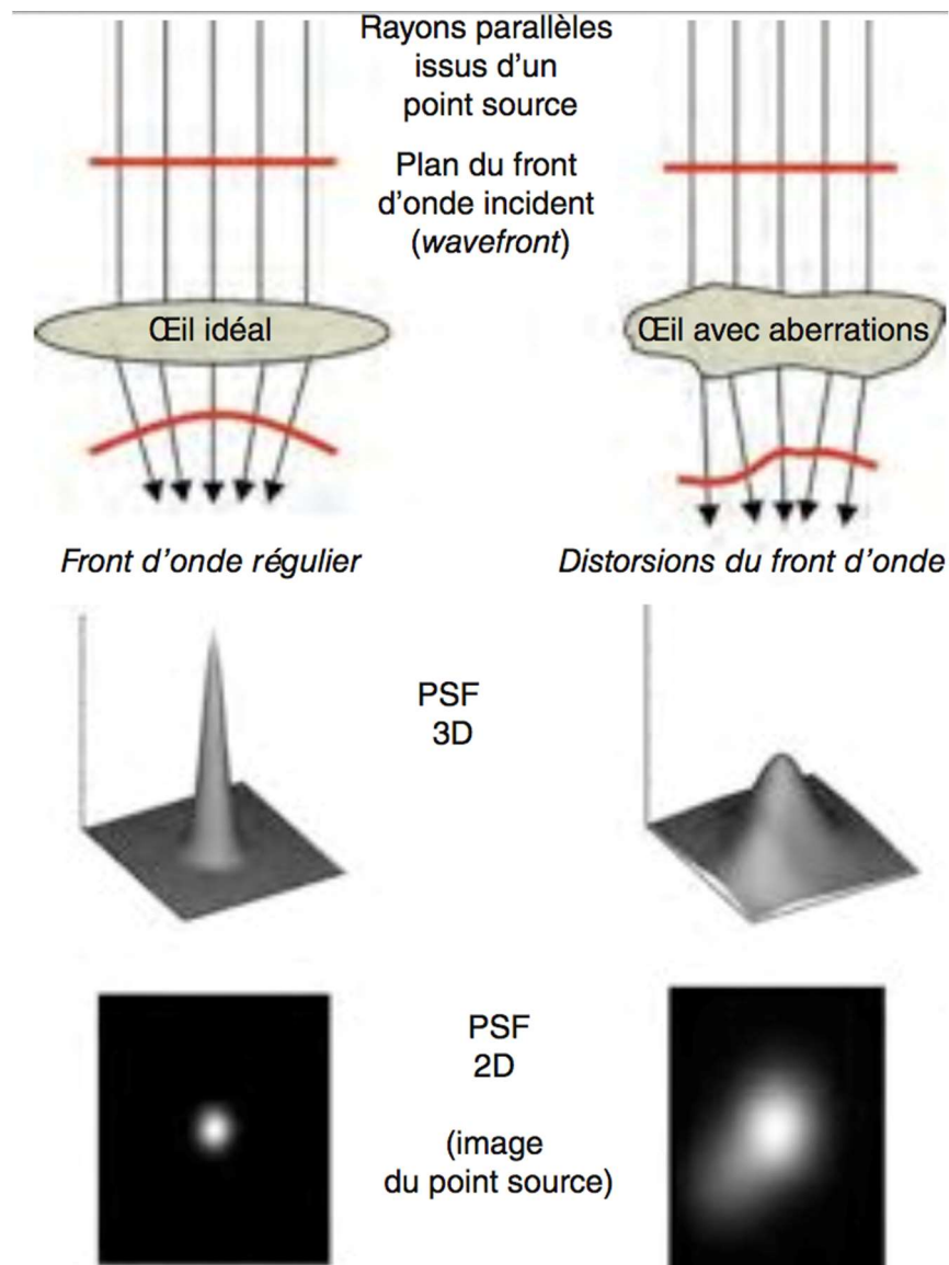
Figure 21 : Principe de l'aberrométrie du front d'onde (Source : Assouline M. (9))
