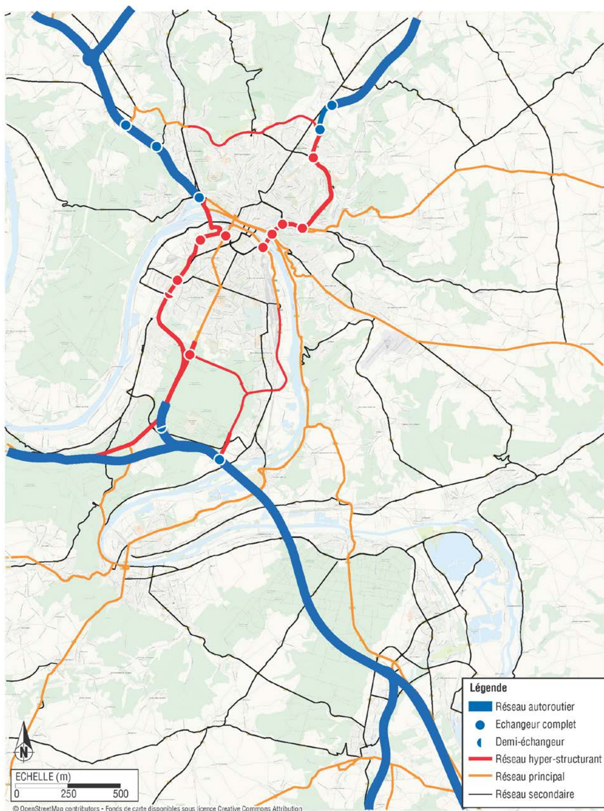
Figure 11 Hiérarchie du réseau routier du secteur de l'agglomération rouennaise réalisée à partir des plateformes de données ouvertes Open Street Map et de SIG puis dessinée avec un logiciel de dessin. Réalisation Transitec Ingénieurs-Conseils
