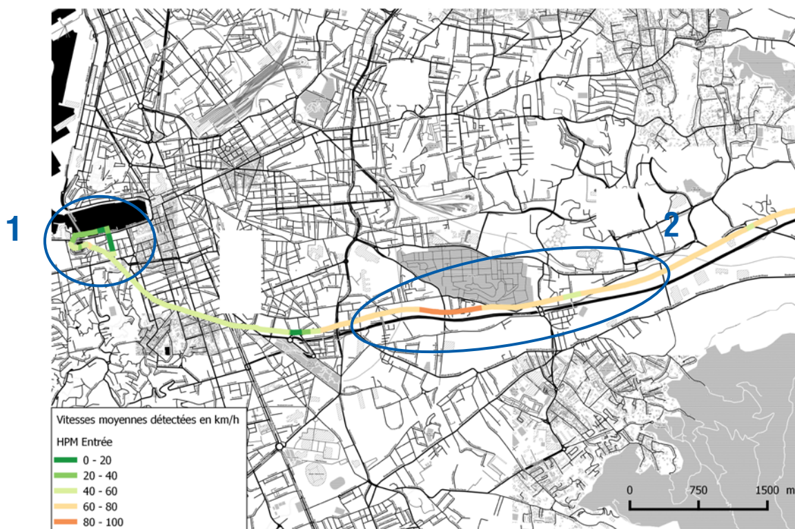
Figure 21 Vitesses moyennes détectées par TOMTOM sur l'A50 en entrée de Marseille en HPM
