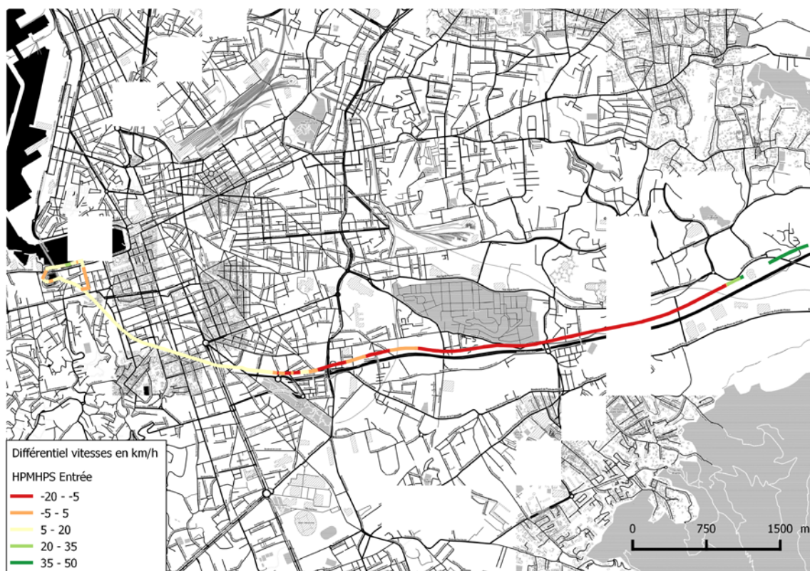
Figure 23 Différentiel des vitesses moyennes détectées en entrée de Marseille par l'A50 en HPM et HPS
