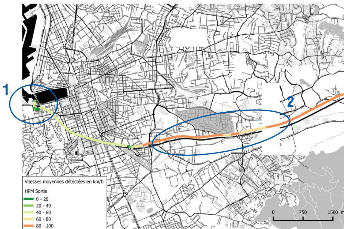
Figure 22 Vitesses moyennes détectées par TOMTOM sur l'A50 en sortie de Marseille en HPM
