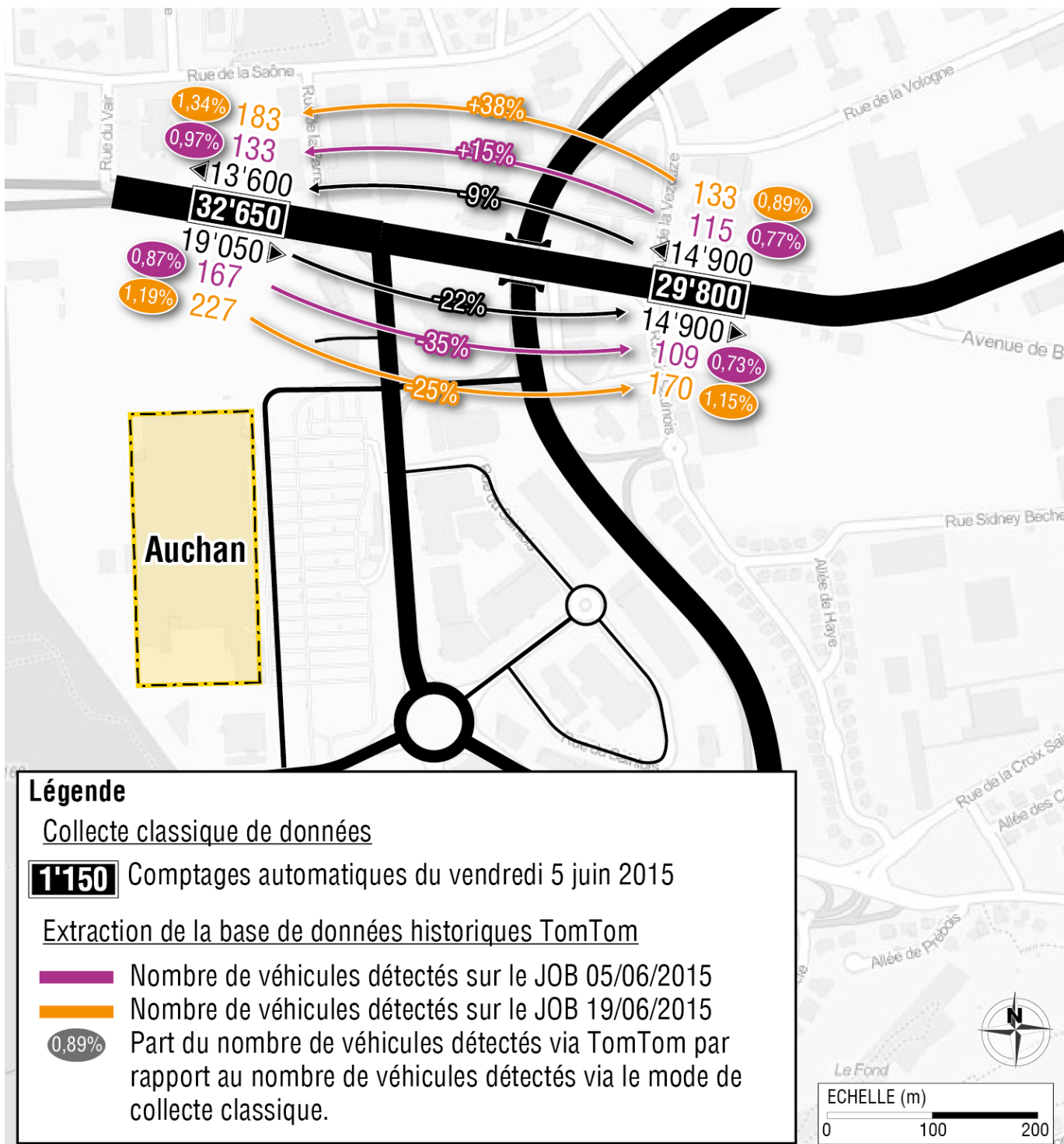
Figure 19 Carte de comparaison des données de comptages obtenues par deux méthodes de collecte de données sur le JOB du vendredi 5 juin 2015
