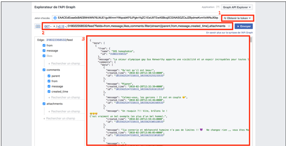
Figure 4 : Capture d'écran de l'API Graph
