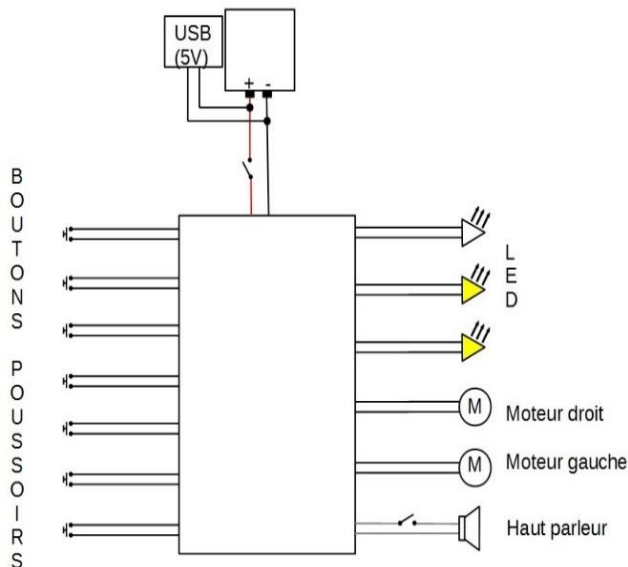
Schéma 1 : carte-mère de la Bee-Bot
