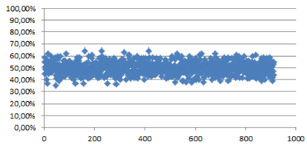
Fréquences de garçons simulées pour des villes de 10000 habitants
