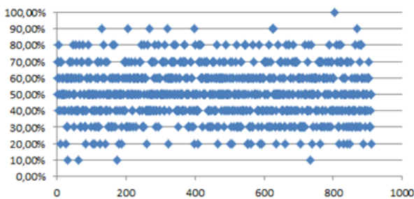
Fréquences de garçons simulées pour des villages de 10 habitants
