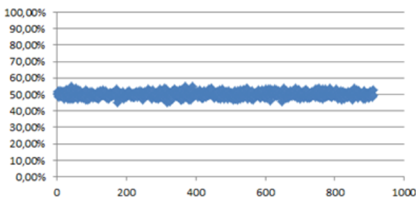
Fréquences de garçons simulées pour des villages de 1000 habitants
