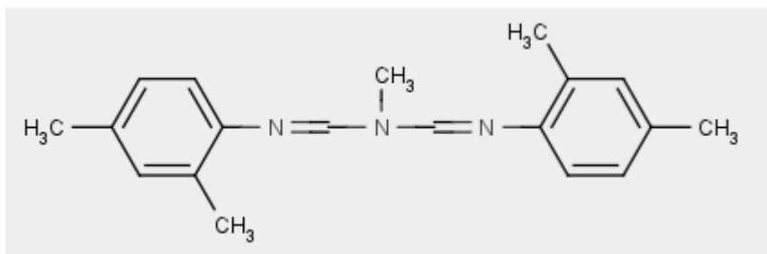
Figure 56 : l'amitraz
