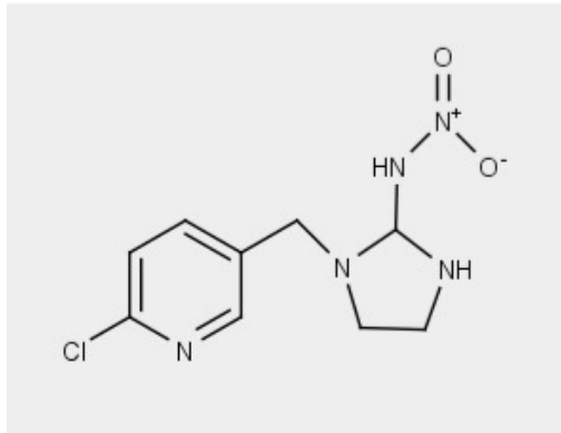
Figure 59 : l'imidaclopride
