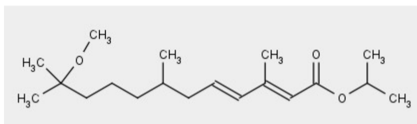
Figure 61 : le S-méthoprène
