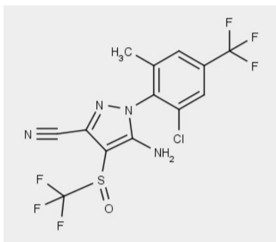
Figure 57 : Le fipronil
