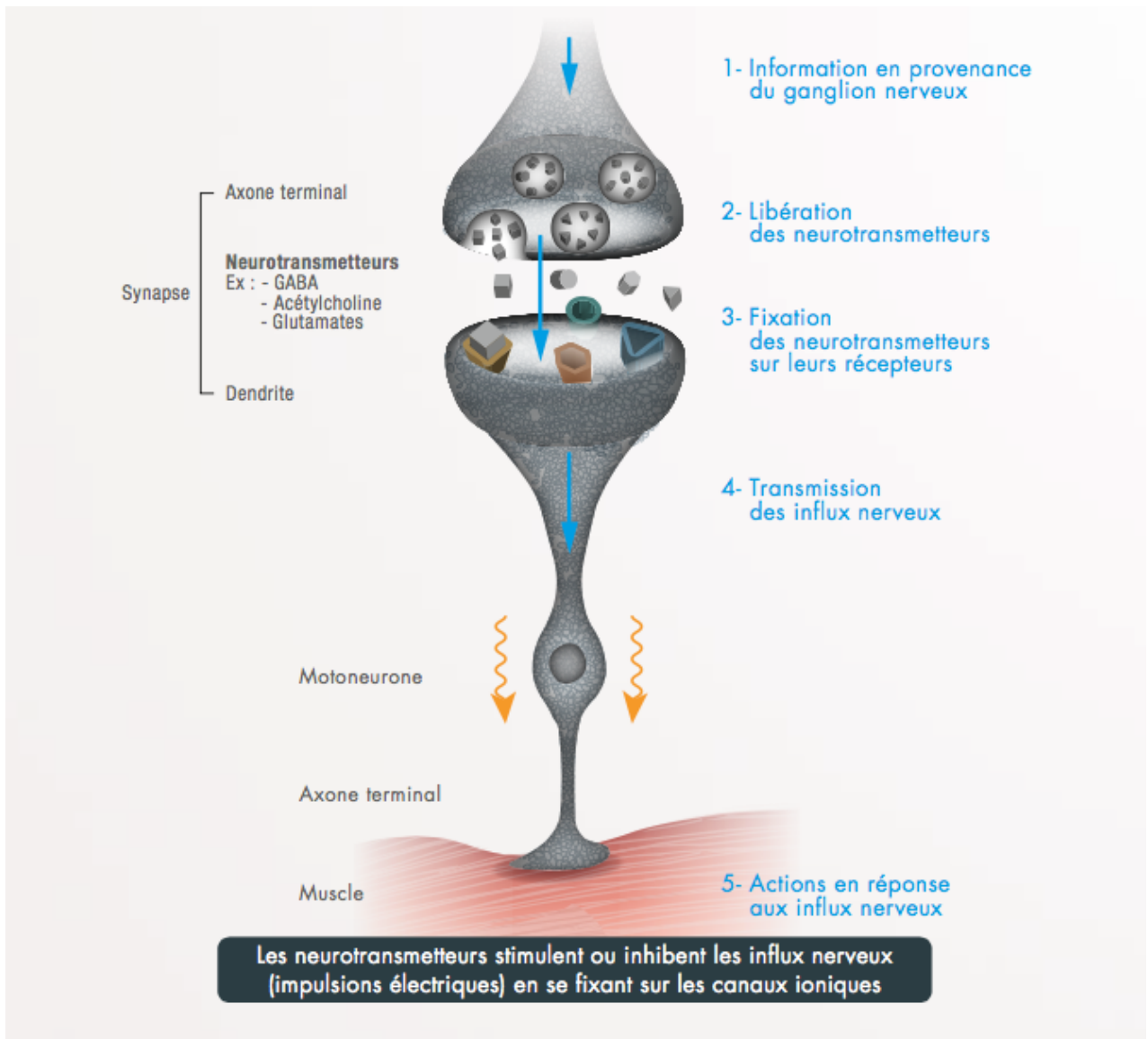
Figure 65 : fonctionnement normal du système nerveux chez les arthropodes (MERIAL, Profil technique Nexgard®, 2014)
