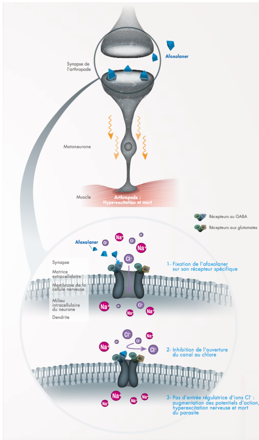
Figure 66 : mode d'action de l'afoxolaner : Inhibition des canaux chlore régité par le GABA (MERIAL, Profil technique Nexgard®, 2014)
