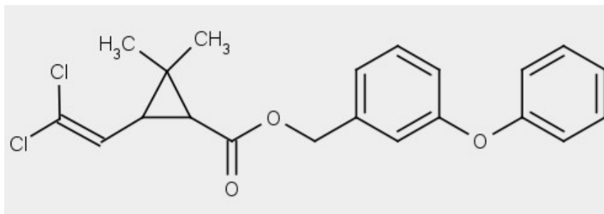
Figure 54 : la perméthrine, pyrèthrinoides de 2 ème génération, largement dominante sur le marché
