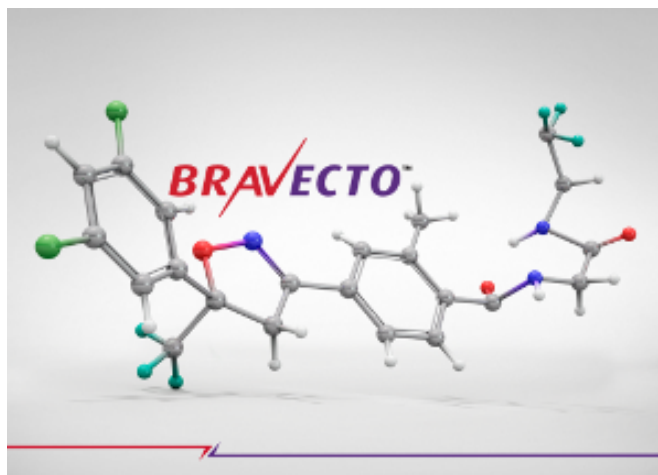
Figure 68 : Le fluralaner
