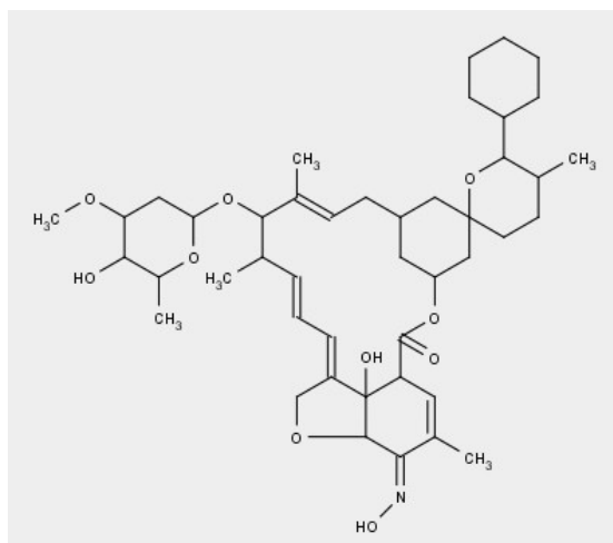
Figure 60 : la sélamectine
