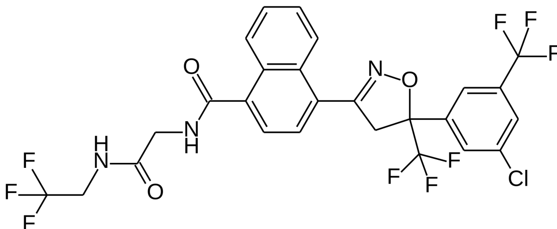
Figure 64 : structure moléculaire de l'afoxolaner
