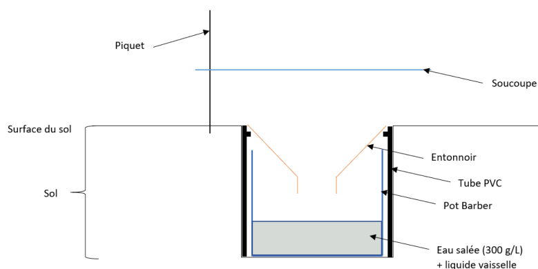
Figure 2 - Schématisation d'un piège Barber (SoilServ 2018)
