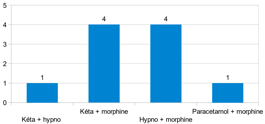
Graphique 6 : Co-prescription d'analgésie-sédation
