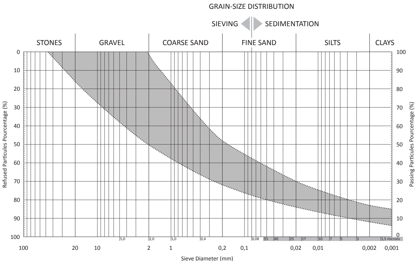
Spectre granulométrique du pisé: traité de construction en terre, Hubert Guillaud et Hugo Houben, éditions Parenthèses, 1989.
