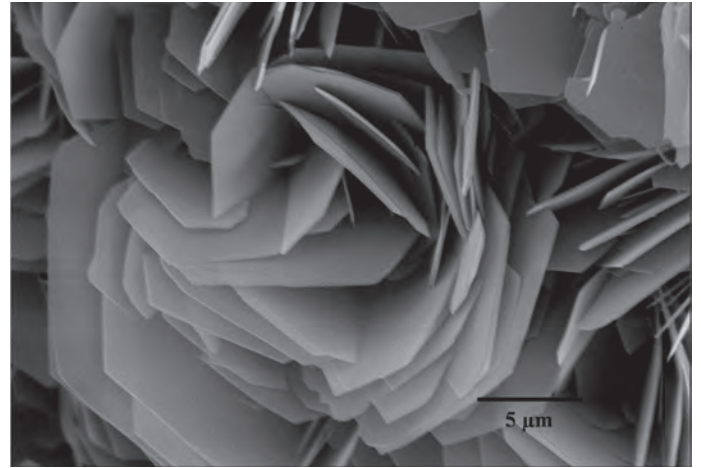
ensemble de plaquettes d'argiles (source bâtir en terre)
