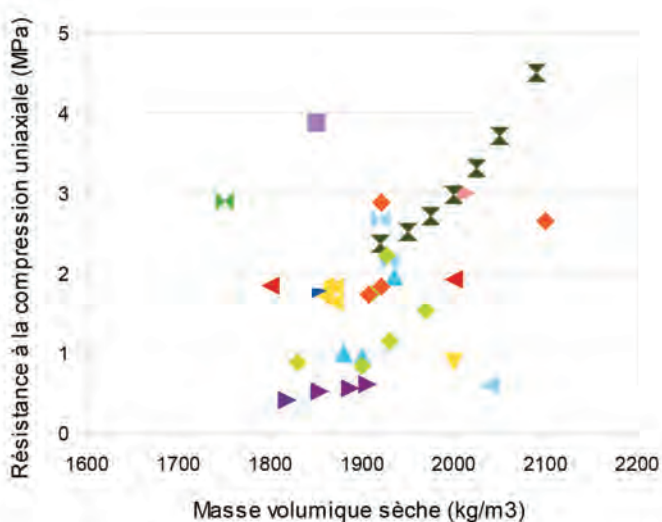
Courbe montrant la relation masse volumique sèche et résistance à la compression, extrait du C2D2
