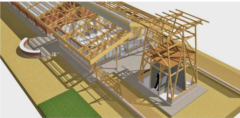
Vue en 3d de la cuisine et la toilette
