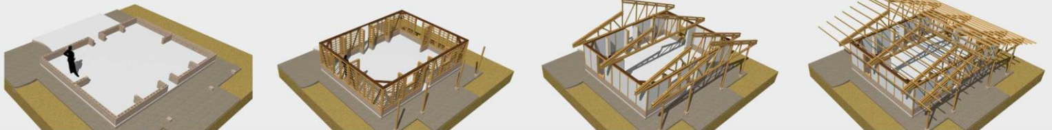
Évolution du système constructif en Torchis / l'espaces de la cuisine
