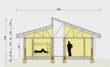
Coupe chambres
