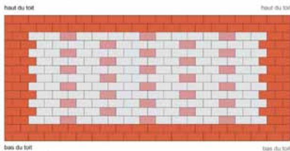
PLAN DE FIXATION DES TUILES EN TOITURE
