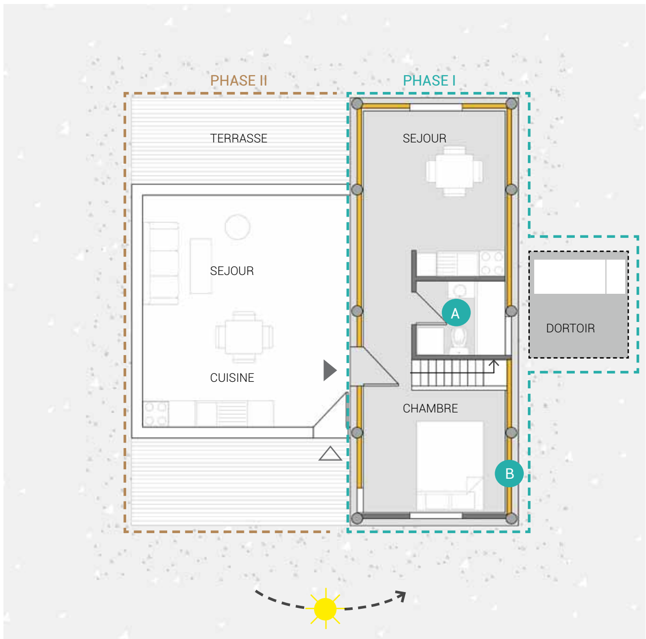
Figure: Plan de la maison à La Floresta-Uruguay. Source: réalisation propre
