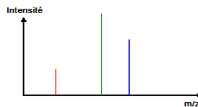
Figure 62 : Diagramme de fragmentation
