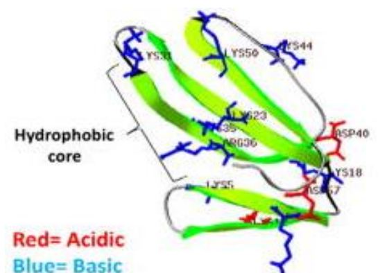
Figure 48 : Structure d'une cardiotoxine III extraite de Naja naja atra .
