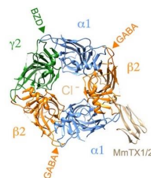
Figure 83: Schéma d'un récepteur GABA A en interaction avec une Micurotoxine [233].
