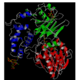
Figure 39 : L-amino acide oxydase
