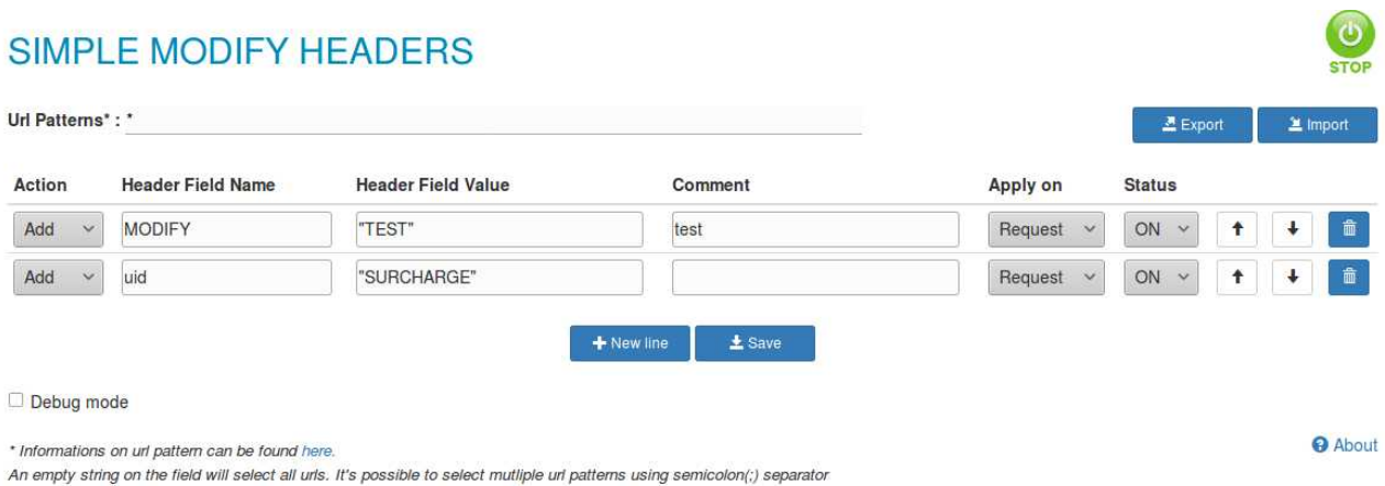
Figure 21 : Entêtes surchargés avec l'extension « ModifyHeaders »
