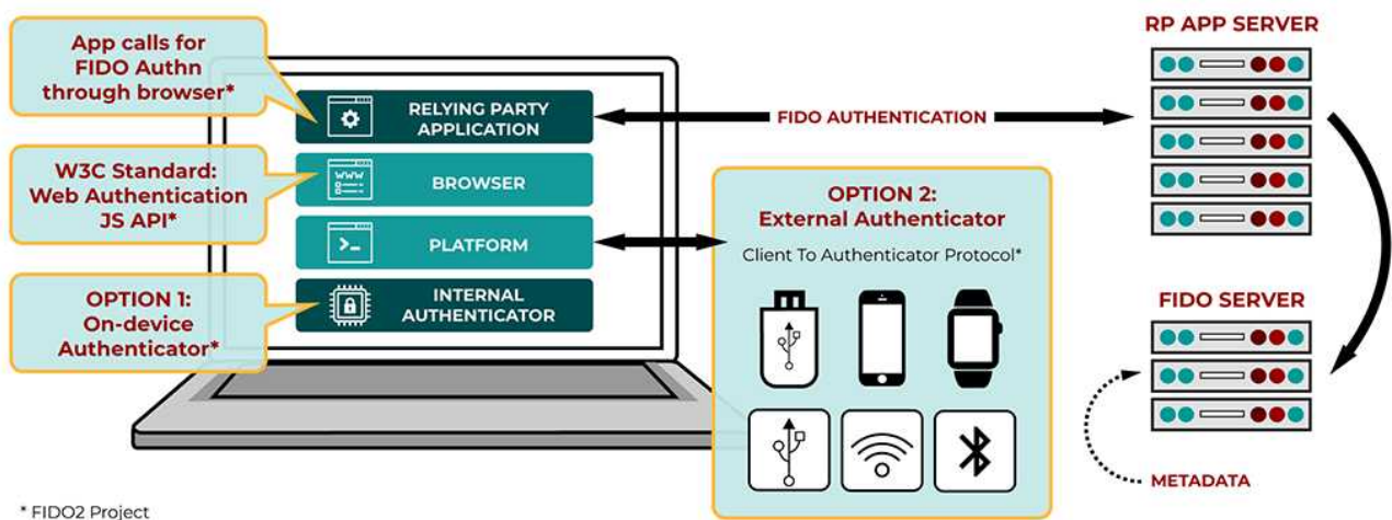
Figure 36 : Norme WebAuthn FIDO-2
