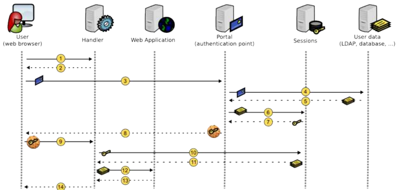
Figure 8 : Cinématique du contrôle d'accès
