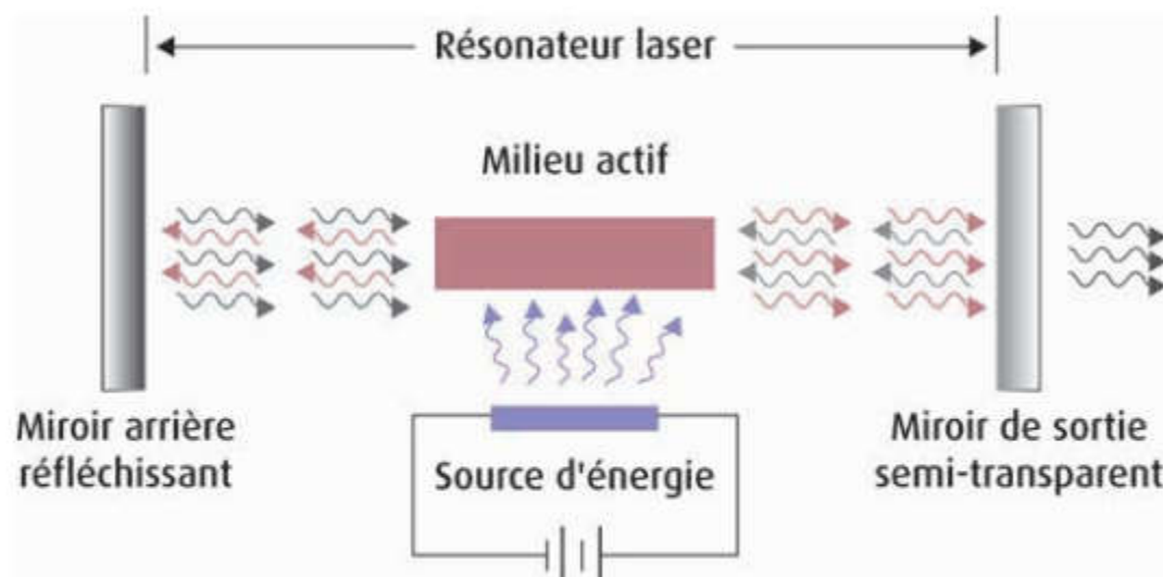
Figure 3 : schéma du laser (20)
