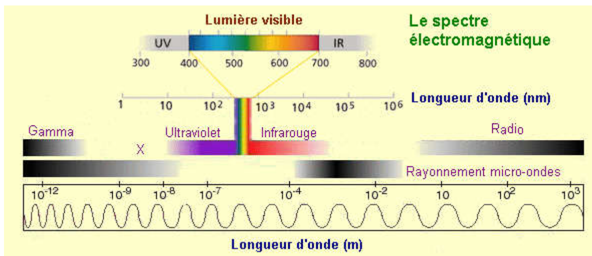
Figure 1 : schéma du spectre électromagnétique et décomposition de la lumière blanche (31)
