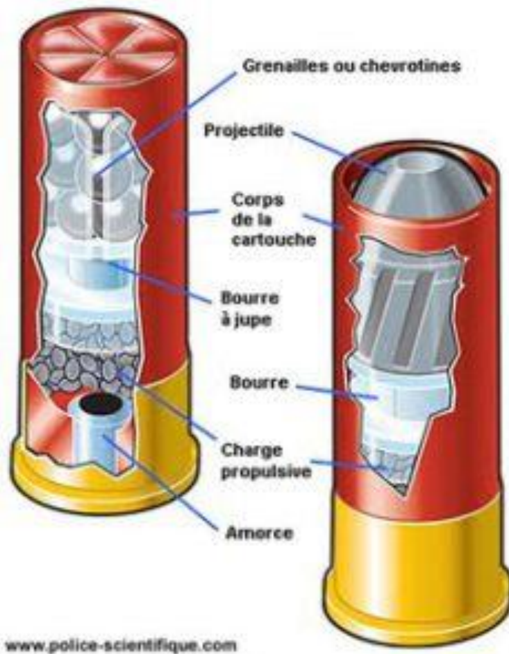
Figure 6: exemple de composition d'une cartouche pour arme à canon lisse
