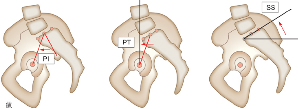
Figure 2 : Paramètres pelviens
