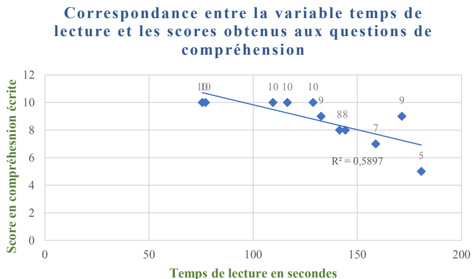
Graphique 6 – Correspondance entre la variable temps de lecture et les scores obtenus aux questions de compréhension.
