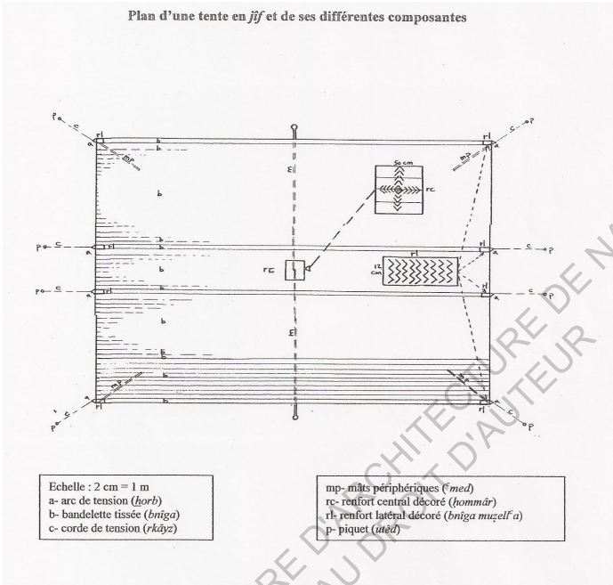
Fig 26. Plan d'une tente en jif et de ses différentes composantes
