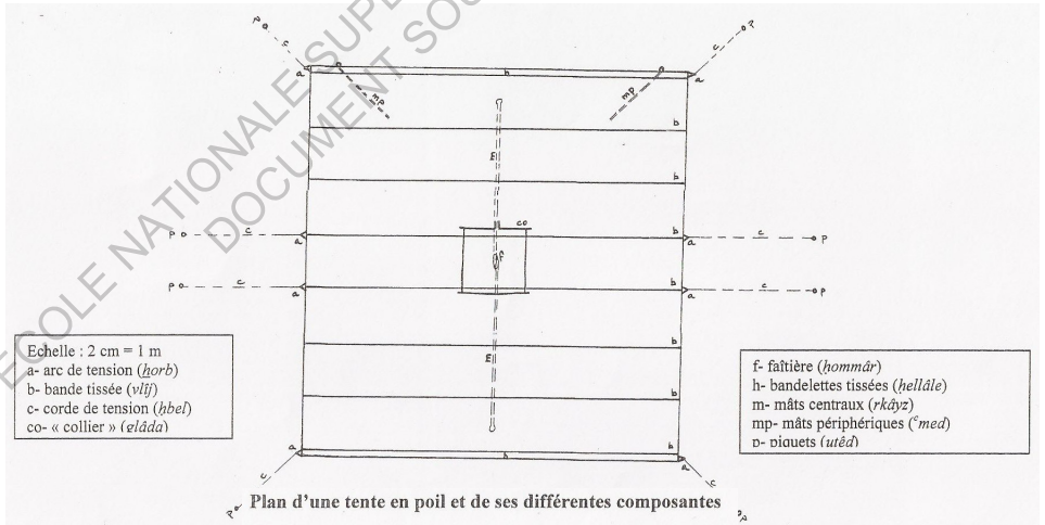
Fig 27. Plan d'une tente en poil et de ses différentes composantes
