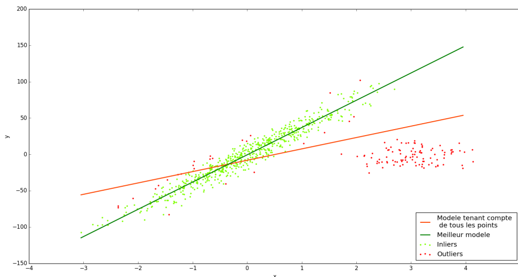
Illustration 13: Principe de l'algorithme RANSAC pour la détection d'une droite dans un espace en deux dimensions (python)
