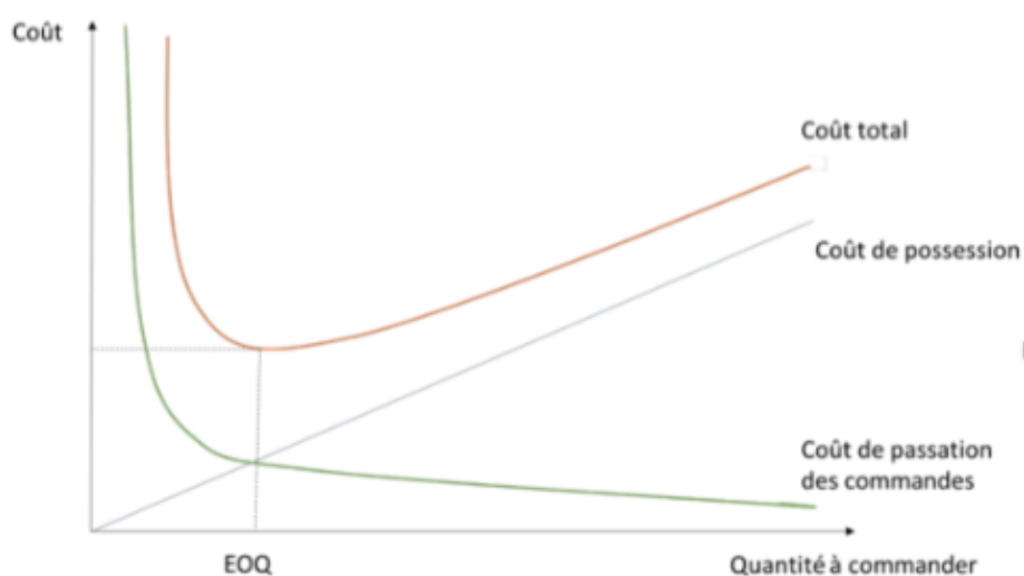
Figure 1 : Détermination de l'EOQ par optimisation du coût total à partir de la méthode de Wilson
