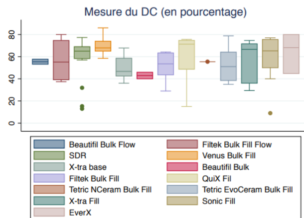
Graphique 3 : Boite à moustache de la distribution des valeurs de DC par composite (bord supérieur de la boite à moustache = troisième quartile, bord inférieur = premier quartile, ligne centrale = médiane, points = valeurs extrêmes)
