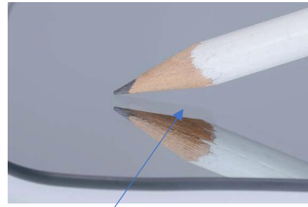
Figure 16 : Image fantôme sur un miroir conventionnel (métallisation sur la face arrière)
