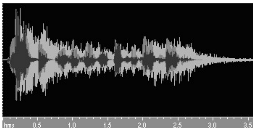
Figure VIII : signal avec 2,0 secondes de temps de réverbération (source : http://www.mcsquared.com/y-reverb.htm )
