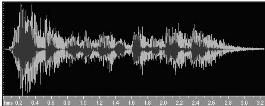
Figure VII : signal avec 1,3 secondes de temps de réverbération (source : http://www.mcsquared.com/y-reverb.htm )
