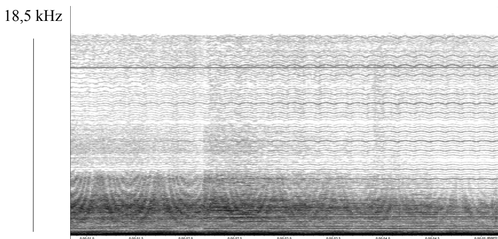
Figure II : les cinq premières secondes du morceau « The Unknown Kadath In The Cold Waste » (Thergothon, 1994)
