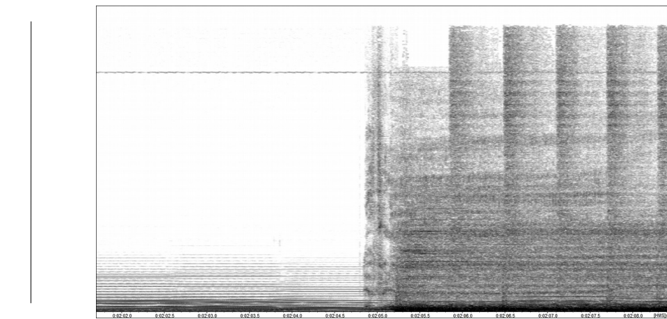
Figure V : « The Rising of the Flames » (Skepticism, 1995) de 2min02 à 2min08.
