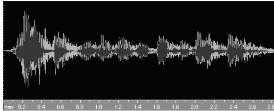
Figure VI : signal avec 0,8 secondes de temps de réverbération (source : http://www.mcsquared.com/y-reverb.htm )
