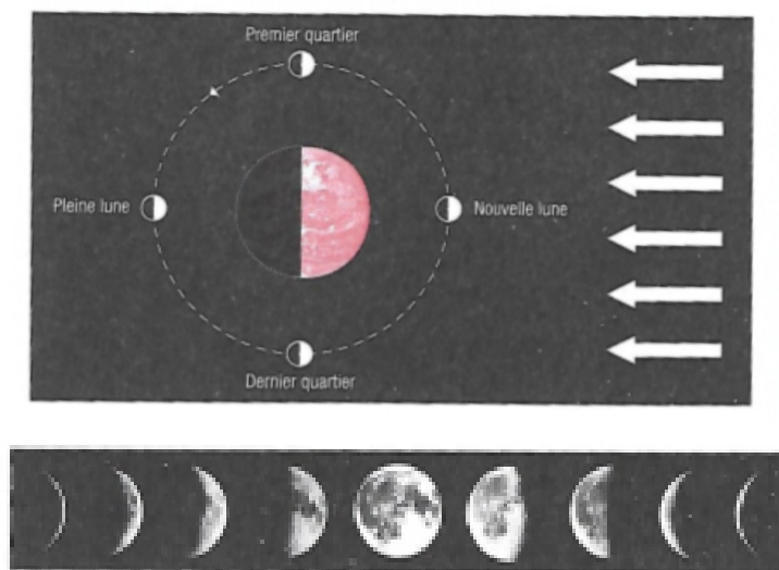
Schémas explicatifs des différentes phases de la Lune 1
