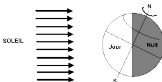
Schéma explicatif de l'alternance jour/nuit 2
