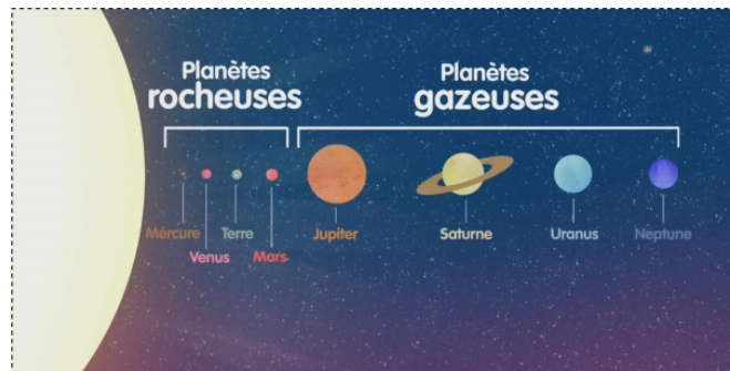
Schéma représentant le système solaire
