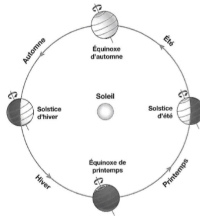
Schéma explicatif de l'alternance des saisons 1
