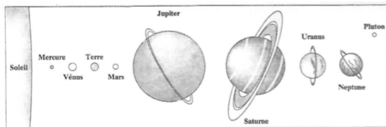
Présentation des planètes du système solaire 1
