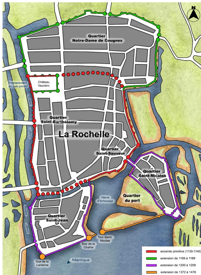
Plan évolutif des fortifications et des différents quartiers de La Rochelle 7
