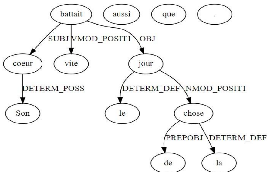
Figure 6 : Exemple de l'ALR
