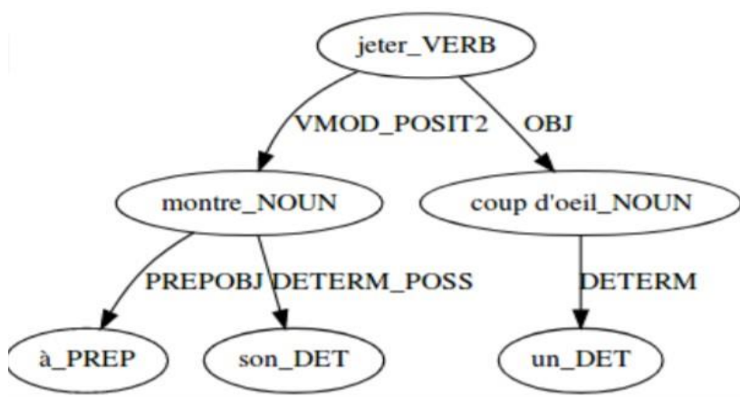
Figure 1 : Exemple d'arbre lexico-syntaxique récurrent (ALR)
