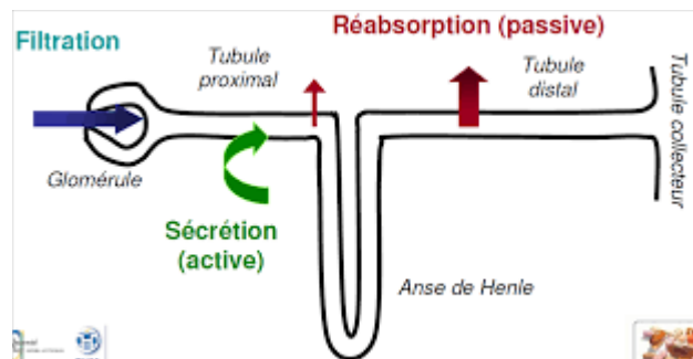
Illustration 32: Schéma de l'élimination rénale des médicaments
