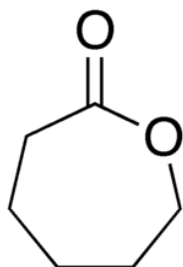
Illustration 25: Structure chimique d'un lactone
