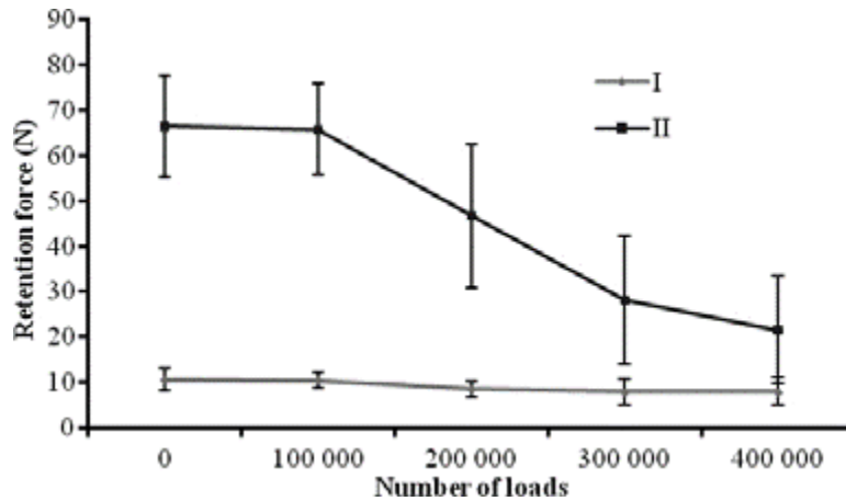
Figure 13 : Evolution de la force de rétention des attachements boule (I) et Locator® (II) en fonction du nombre de cycles de mastication (Abi Nader et al. 2011).
