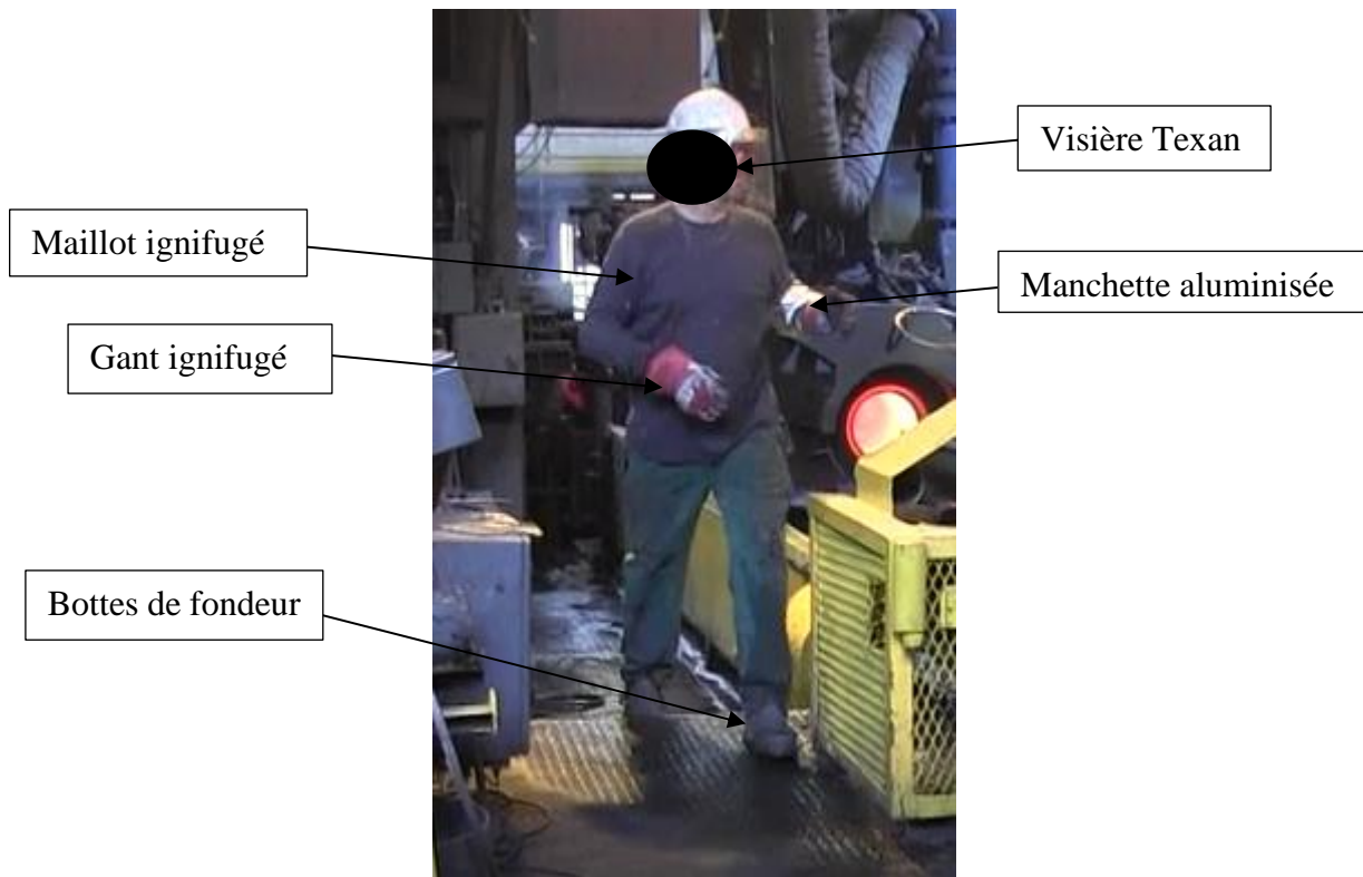
Photo 1 : Port de vêtements ignifugés lors d'une opération d'écrouissage du basket
