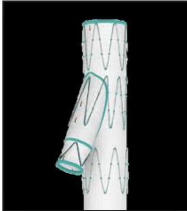
Figure 1 : Endoprothèse branchée iliaque ZBIS (Cook®)
