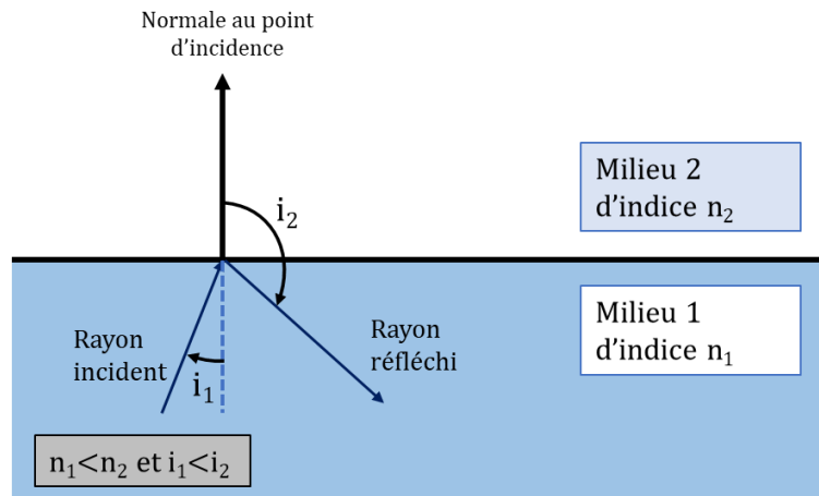
Figure 8 : Réflexion totale
